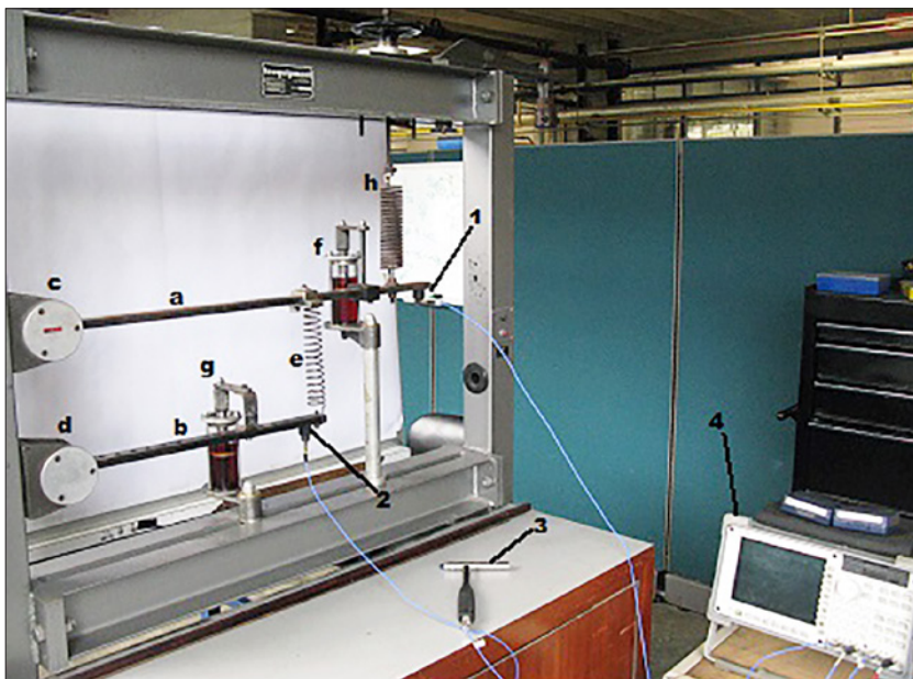
Figura 1. Montaje experimental
