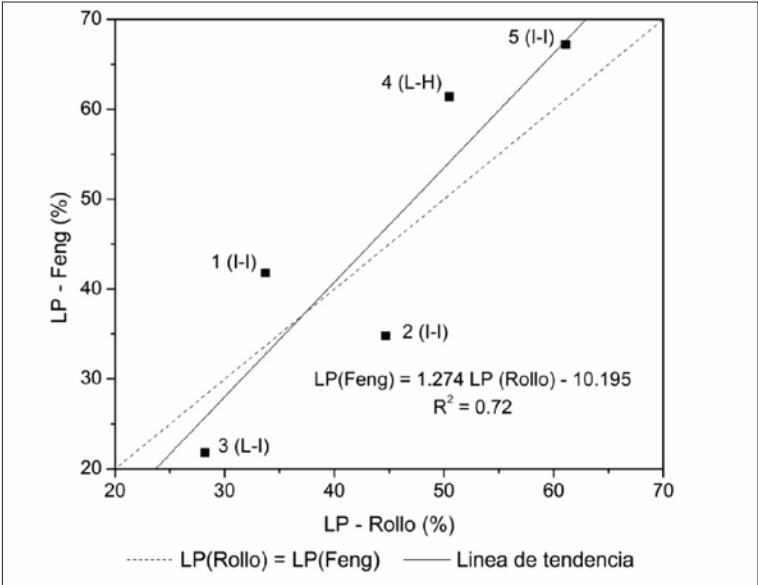
Figura 5. Gráfica de relación entre los límites plásticos según [18] y método de rollo al clasificar los suelos con el nuevo sistema
