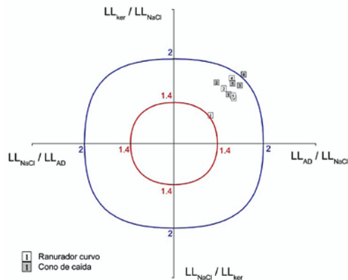
Figura 3. Representación gráfica de la sensibilidad eléctrica de los cinco suelos. Método cono y ranurador curvo.
