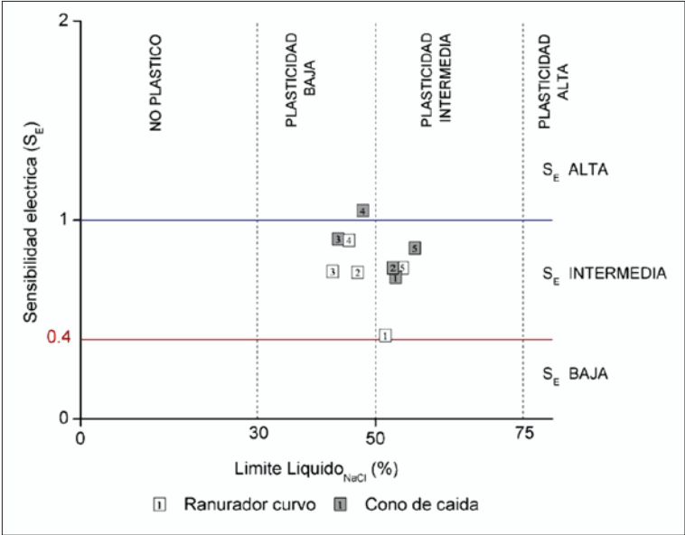
Figura 4. Ubicación de los cinco suelos en la nueva carta de clasificación
