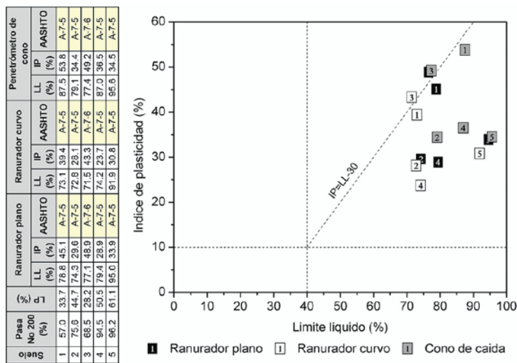
Figura 2. Clasificación AASHTO de las muestras por los tres métodos utilizados (la tabla presenta el resumen de valores).
