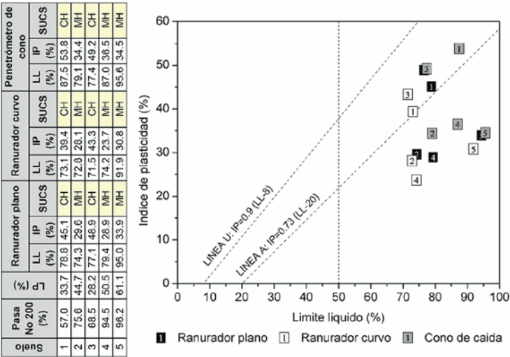
Figura 1. Clasificación SUCS de las muestras por los tres métodos utilizados (la tabla presenta el resumen de valores).
