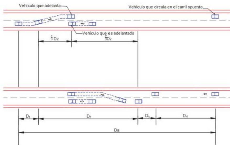
Figura 1 Distancia de Visibilidad de Adelantamiento según la AASHTQ
