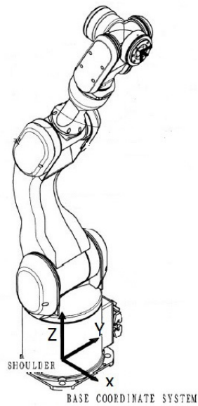
FIGURA 9. EJES CARTESIANOS DEL LEAP MOTION VERSUS ESTRUCTURA FÍSICA DEL PA10.
