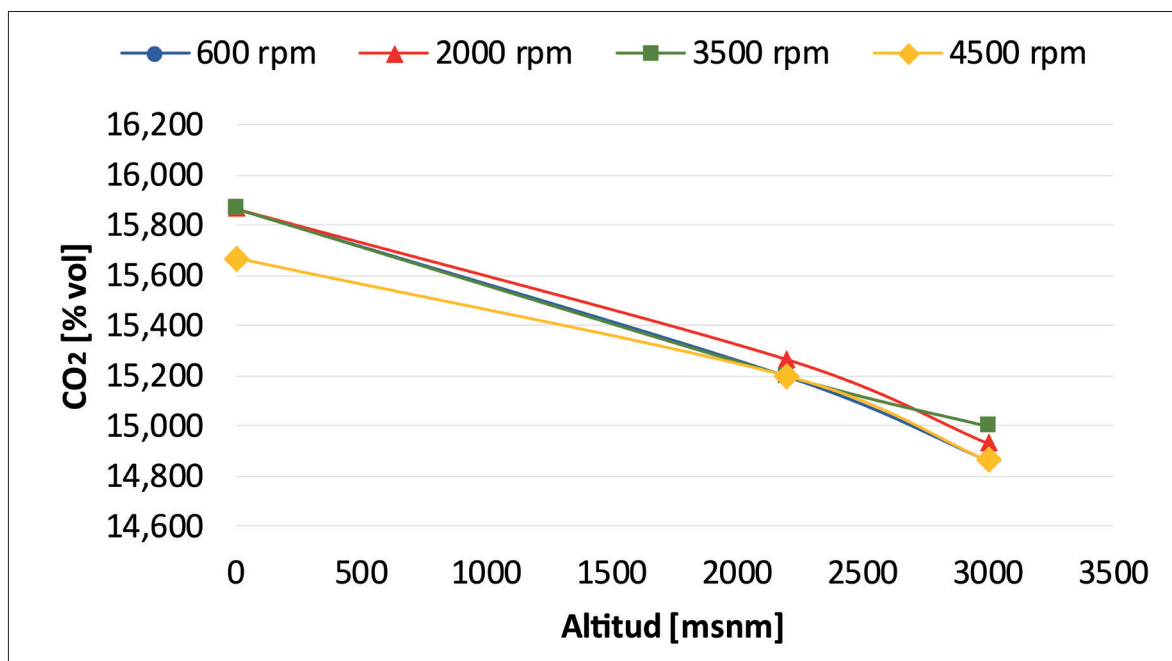
FIGURA 4. EFECTO DE LA ALTITUD SOBRE LAS EMISIONES DE CO 2
