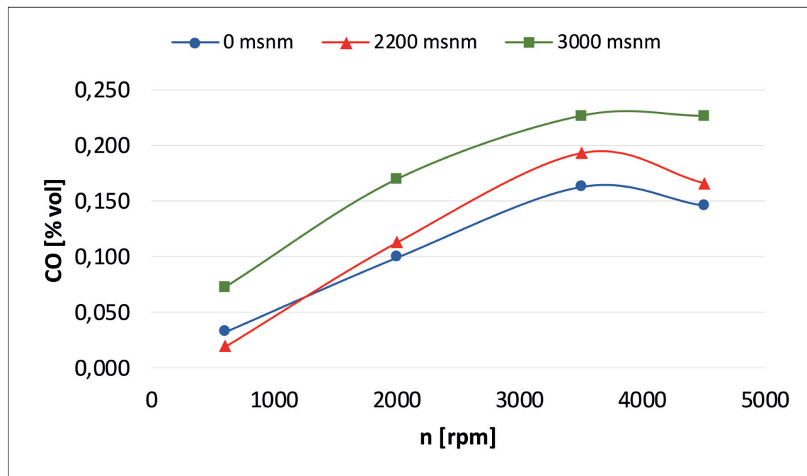
FIGURA 3. EFECTO DE LAS REVOLUCIONES DEL MOTOR SOBRE LAS EMISIONES DE CO
