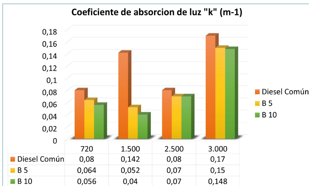
FIGURA 2. COEFICIENTE DE ABSORCIÓN DE LUZ POR RPM CON CADA COMBUSTIBLE
