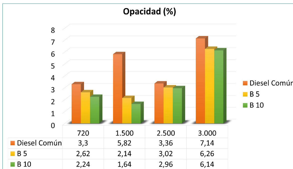
FIGURA 1. PORCENTAJE DE OPACIDAD POR RPM CON CADA COMBUSTIBLE
