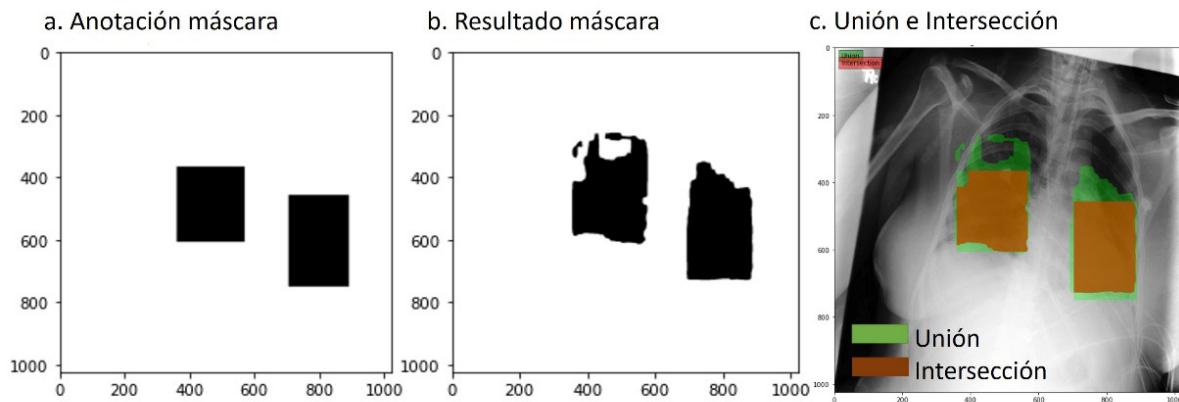
FIGURA 4. APLICACIÓN DE LA MÉTRICA IoU INDIVIDUAL: A. ANOTACIÓN MÁSCARA, B. RESULTADO MÁSCARA, C. UNIÓN E INTERSECCIÓN
