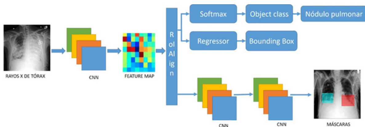
FIGURA 1. MODELO BASADO EN MASK-RCNN PARA IDENTIFICACIÓN DE OPACIDAD PULMONARES
