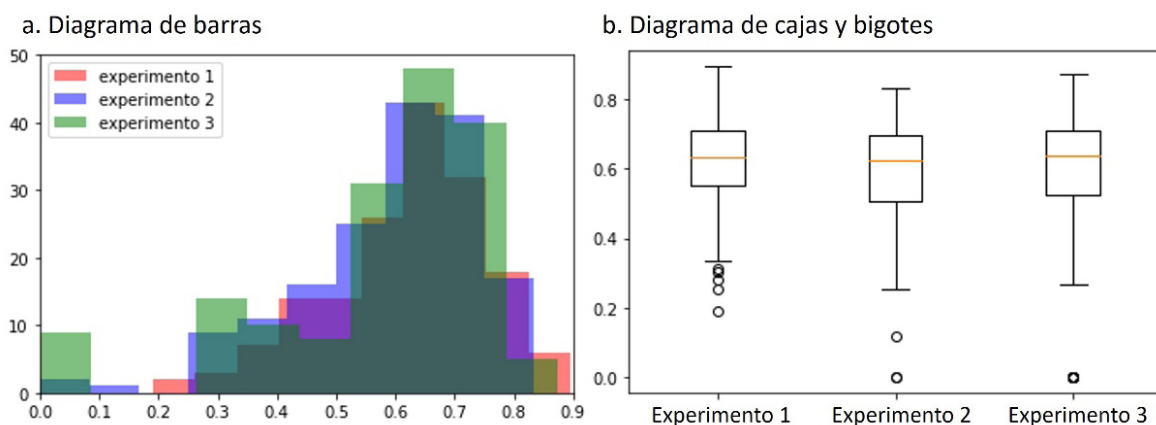
FIGURA 5. DIAGRAMAS DE DESEMPEÑO DE LA MÉTRICA IoU GLOBAL DE GRUPO DE IMÁGENES TEST
