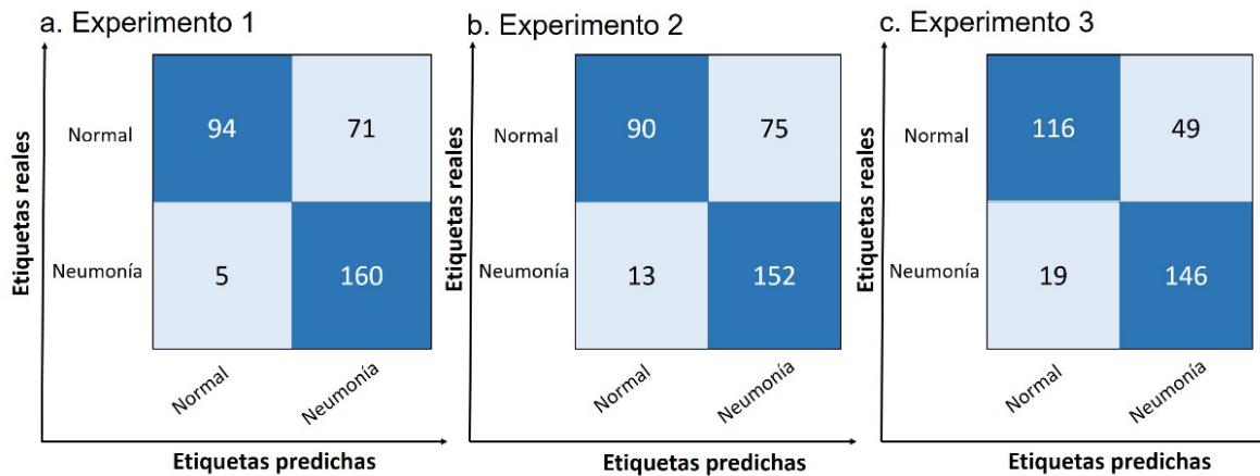
FIGURA 6. MATRIZ DE CONFUSIÓN DE LOS EXPERIMENTOS: A. EXPERIMENTO 1, B. EXPERIMENTO 2, C. EXPERIMENTO 3
