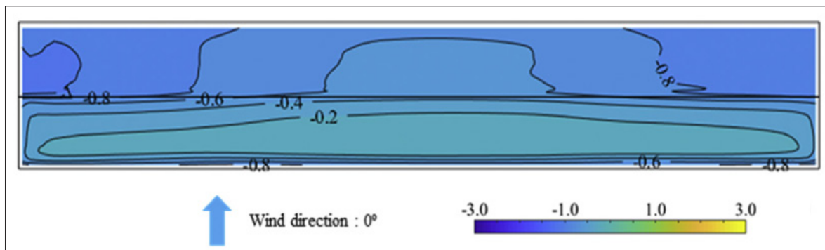
FIGURA 7. CONTORNO DE DISTRIBUCIÓN DE PRESIONES EN EDIFICACIÓN (VI) CON CUBIERTA DE INCLINACIÓN 22^\circ (TÚNEL DE VIENTO) [19]
