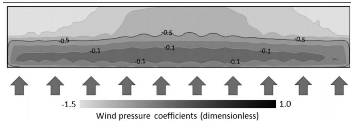
FIGURA 6. CONTORNO DE DISTRIBUCIÓN DE PRESIONES EN EDIFICACIÓN (V) CON CUBIERTA DE INCLINACIÓN 26^\circ [18]
