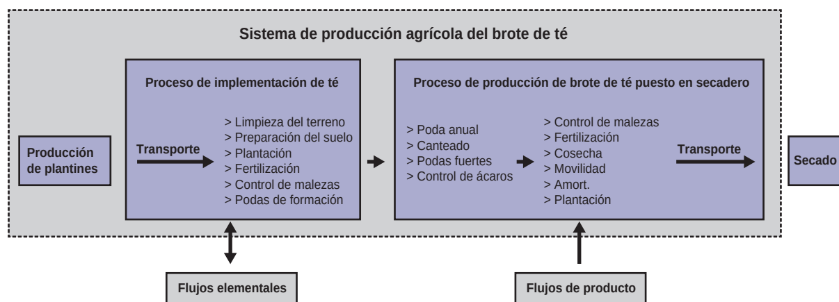
Figura 1. Sistema de producción del brote de té.
