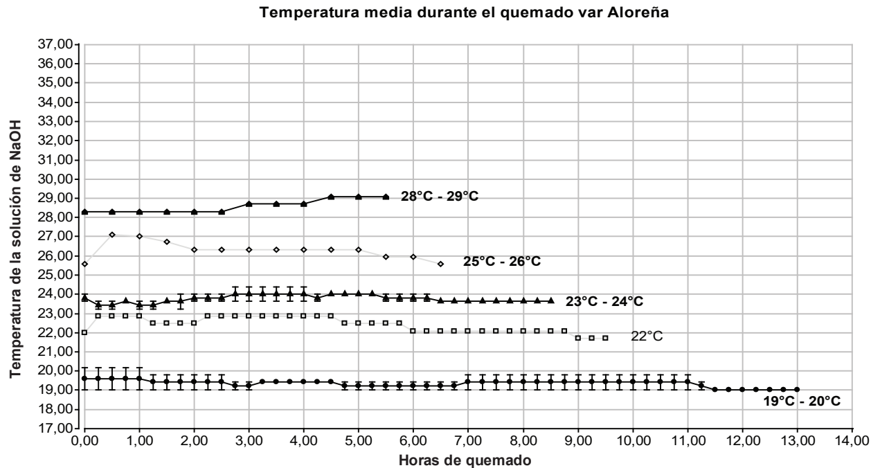
Figura 2. Temperaturas medias y su desviación estándar de los valores registradas en los tratamientos durante el quemado de variedad Aloreña.
