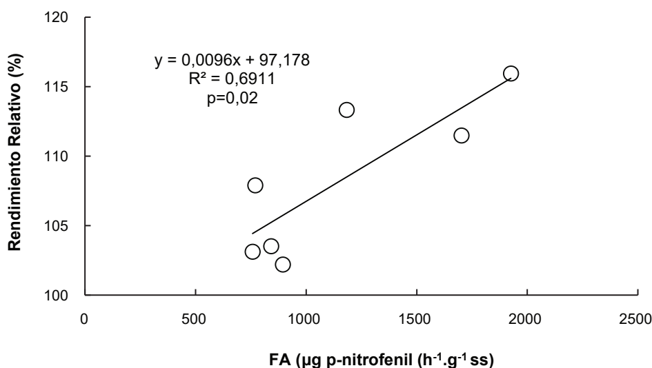
Figura 5. Relación lineal simple entre rendimiento relativo (%) y FA (Fosfatasa ácida, (μg p-nitrofenil h -1 g -1 ss)) teniendo en cuenta las parcelas aplicadas de CC y B correspondientes a las cuatro campañas. La elipse encierra los valores de Vicia (V) y Barbecho (B) de 2016/2017.
