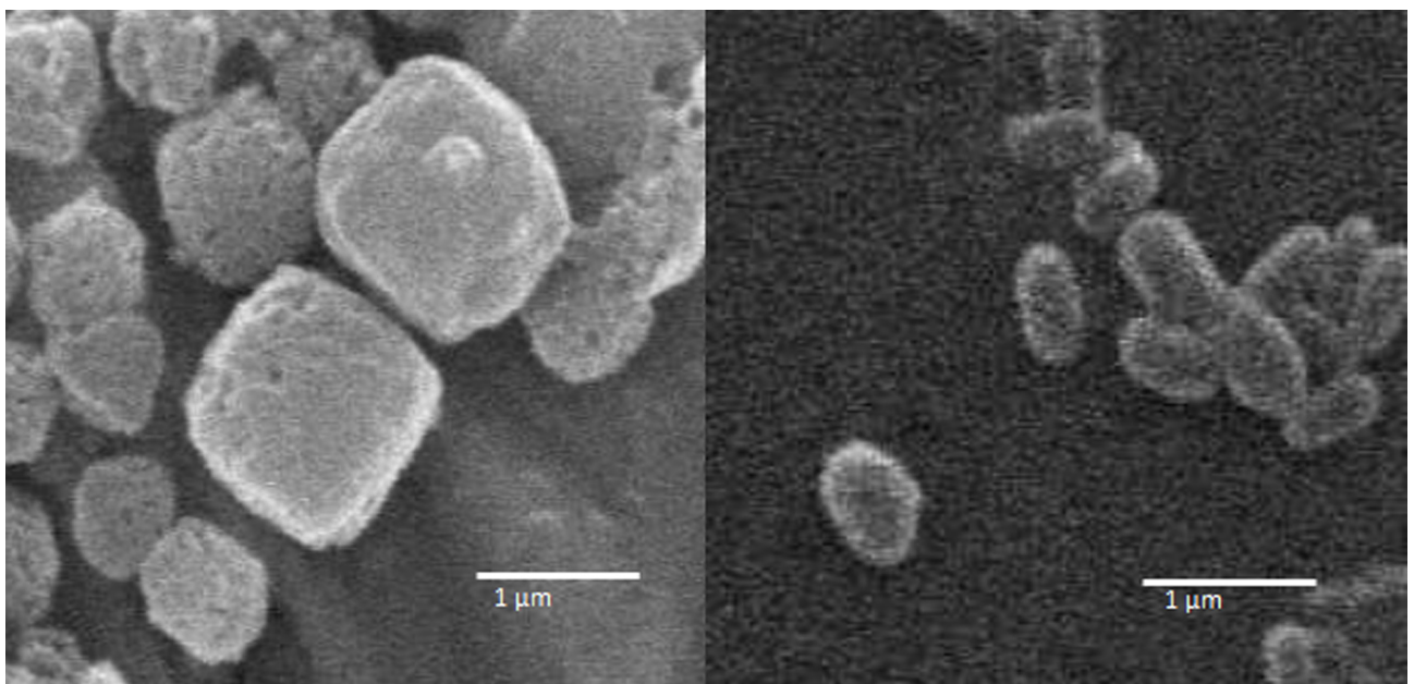
Figura 1. Cuerpos de oclusión baculovirales (OBs). Izquierda: poliedros de Autographa californica Multiplicinucleopoliedrovirus (AcMNPV). Derecha: gránulos de Epinotia aporema Granulovirus (EpaGV). (Fotos obtenidas por microscopía electrónica de barrido. Ricardo Salvador).
