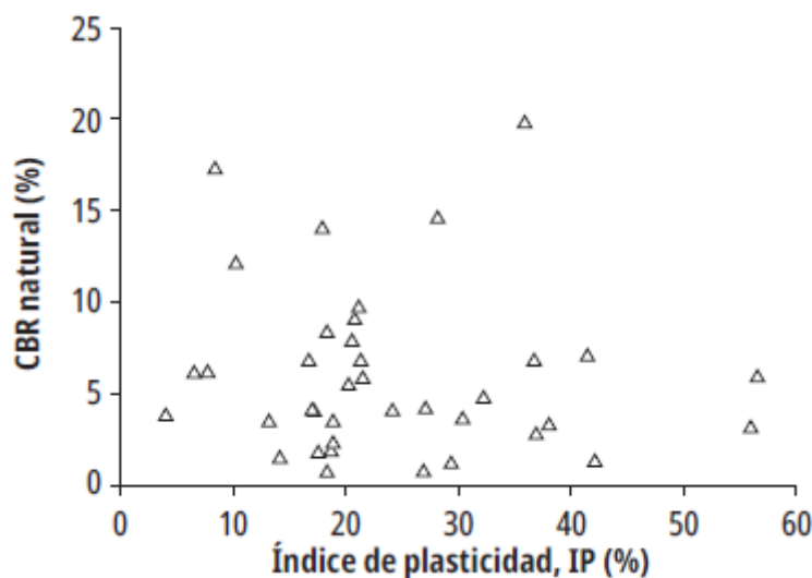
Figura 2 Dispersión CBR natural versus índice de plasticidad. Fuente: Elaboración propia.
