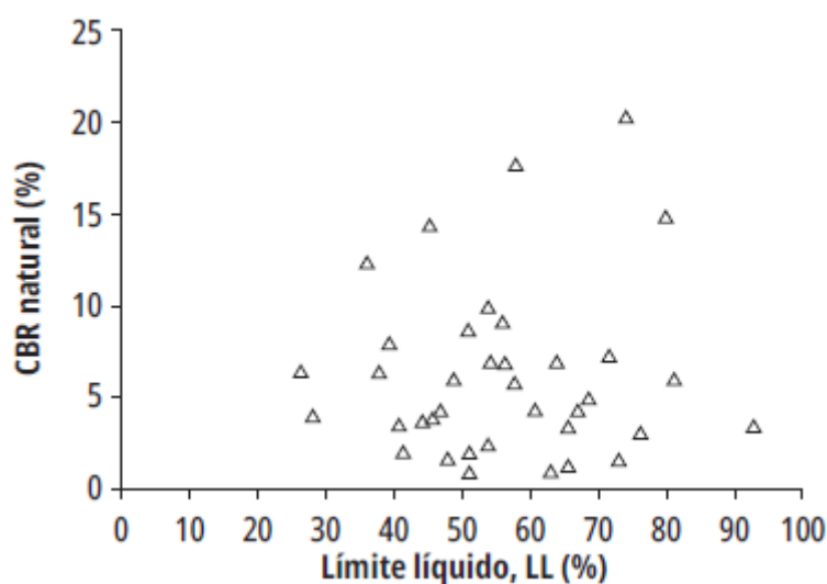
Figura 1 Dispersión CBR natural versus límite líquido. Fuente: Elaboración propia.
