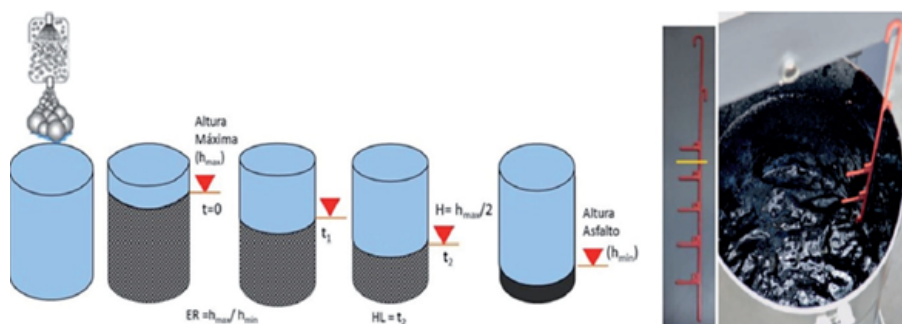
Figura 4 Método de la varilla graduada. Fuente: Elaboración propia.
