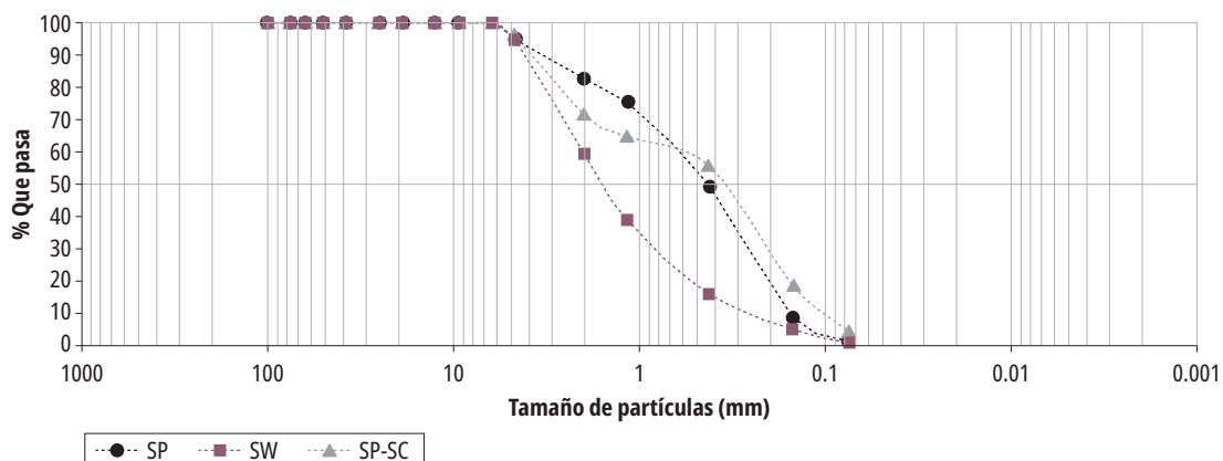
Figura 3. Distribución granulométrica de los materiales empleados en la modelación
