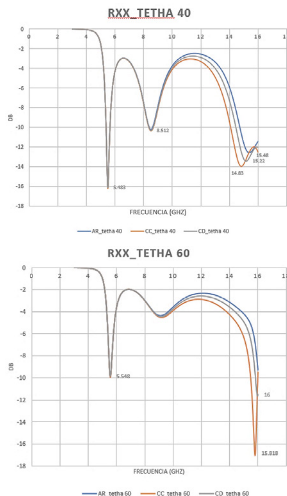
Figura 15. Curva S_{11} de anillo resonador (AR), cruz central (CC) y cruz doble (CD). Incidencia a 40^\circ y 60^\circ
