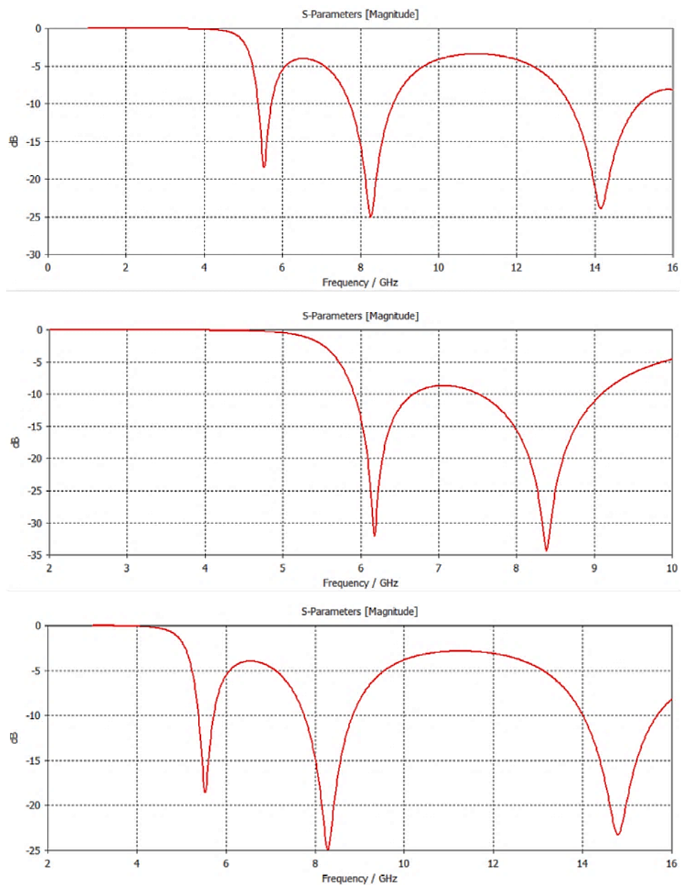
Figura 11. Curvas S_{11} para los tres últimos diseños de celdas unitarias
