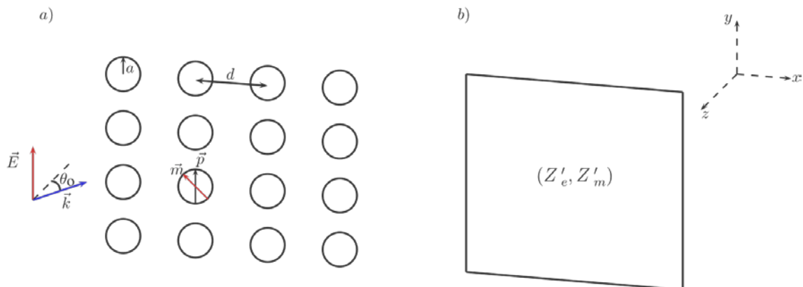
Figura 4. Una metasuperficie denominada metafilm (a) y su caracterización como superficie de impedancia (b)
