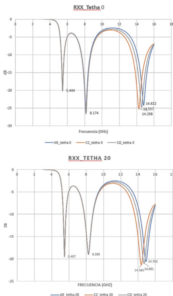
Figura 14. Curva S_{11} de anillo resonador (AR), cruz central (CC) y cruz doble (CD). Incidencia a 0^\circ y 20^\circ
