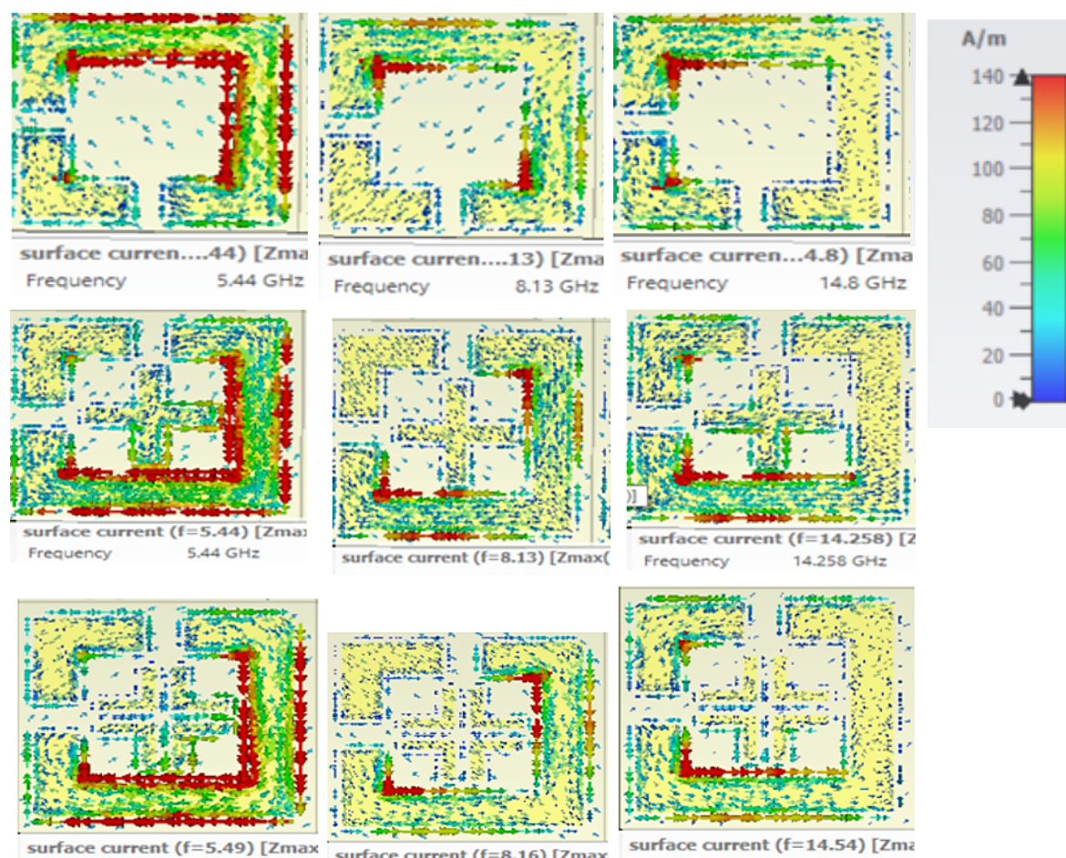
Figura 17. Densidades de corriente para las celdas unitarias estudiadas
