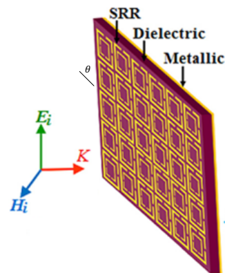
Figura 13. Esquemático de radiación incidente sobre la celda unitaria analizada
