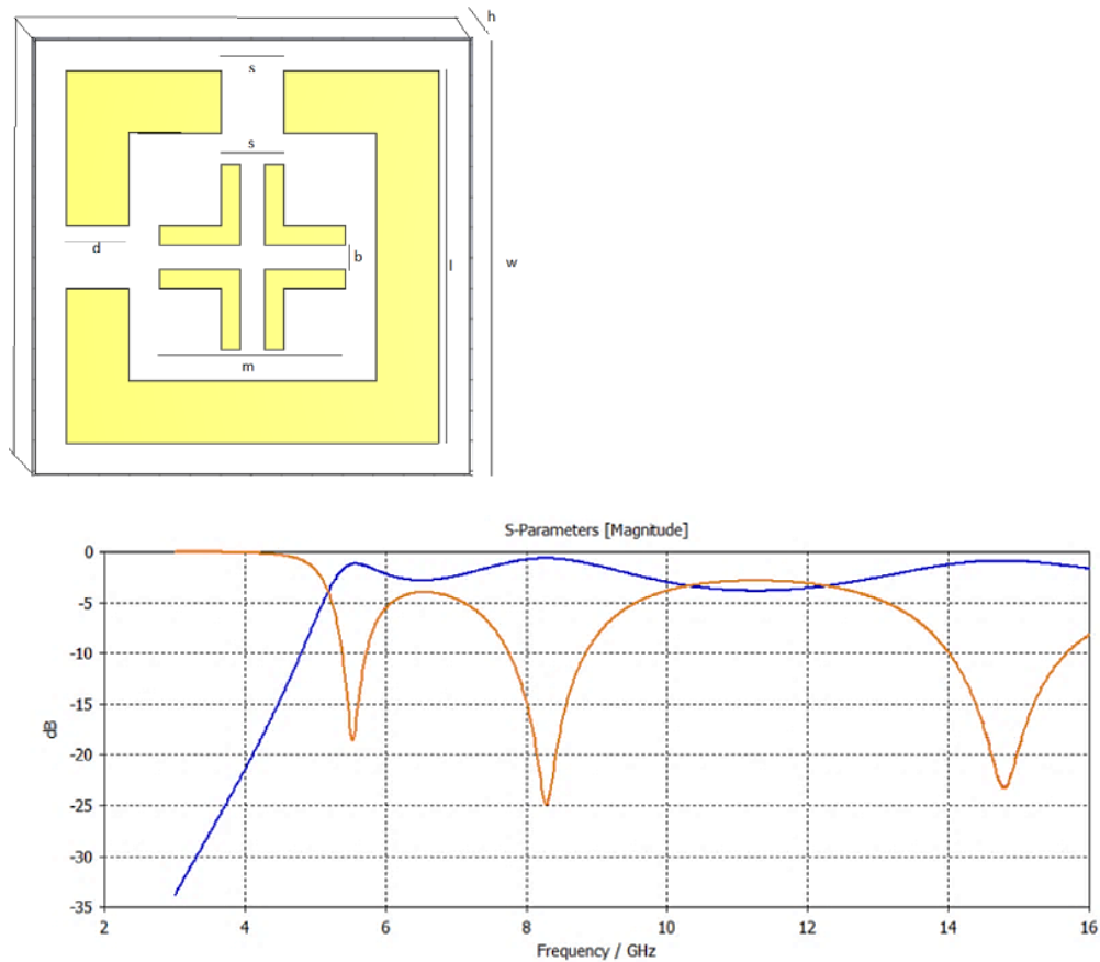
Figura 12. Celda unitaria por analizar de manera detallada y curva S_{12} (azul) de la celda unitaria
