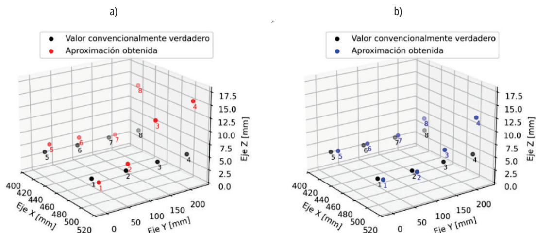
Figura 17. a) Valor convencionalmente verdadero vs valor obtenido en una resolución de ; b) valor convencionalmente verdadero vs valor obtenido en una resolución de 640 x 480
