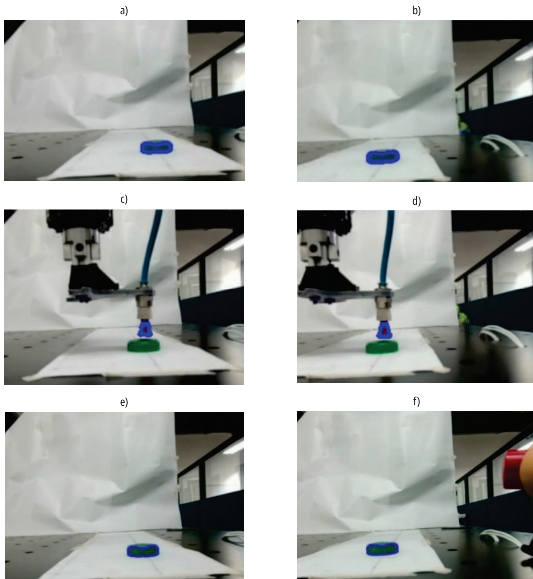
Figura 16. a) Detección de la pieza cámara izquierda, resolución 320x240; b) detección de la pieza cámara derecha, resolución 320x240; c) detección de la ventosa cámara izquierda, resolución 320x240; d) detección de la ventosa cámara derecha, resolución 320x240; e) detección de la pieza cámara izquierda, resolución 640x480; f) detección de la pieza cámara derecha, resolución 640x480; g) detección de la ventosa cámara izquierda, resolución 640x480; h) detección de la ventosa cámara derecha, resolución 640x480; i) detección de la pieza cámara izquierda, resolución 1280x720; j) detección de la pieza cámara derecha, resolución 1280x720; k) detección de la ventosa cámara izquierda, resolución 1280x720; l) detección de la ventosa cámara derecha, resolución 1280x720
