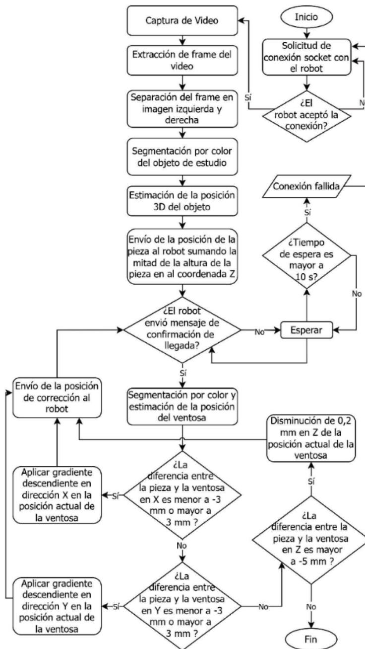
Figura 14. Diagrama de flujo de la corrección de la posición
