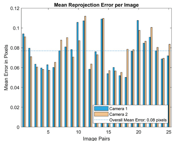
Figura 4. Error medio de proyección por imagen en resolución 320x240 píxeles
