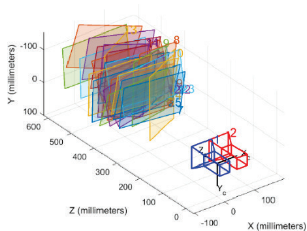
Figura 5. Visualización de parámetros extrínsecos, resolución 320x240 pixeles
