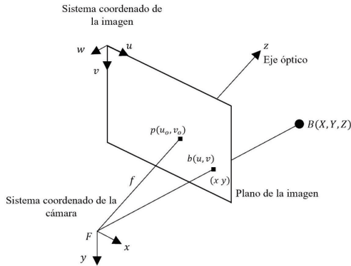
Figura 1. Geometría proyectiva de la cámara estéreo
