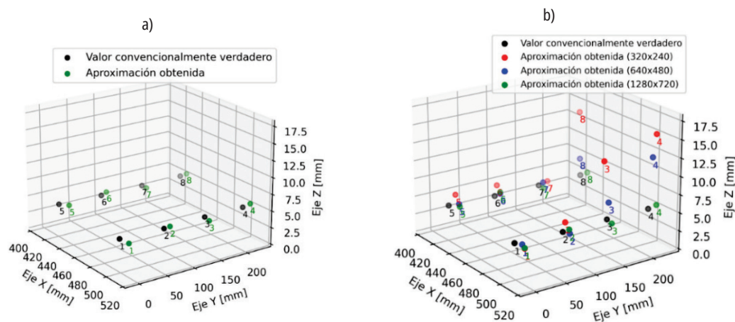
Figura 18. a) Valor convencionalmente verdadero vs valor obtenido en una resolución de 1280x720; b) comparación entre el valor convencionalmente verdadero vs valor obtenido en todas las resoluciones
