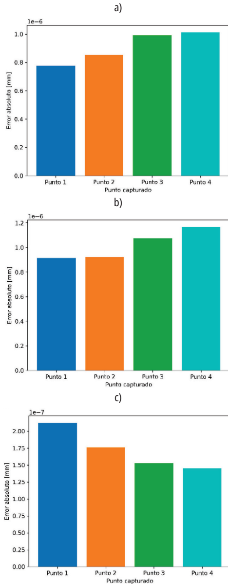
Figura 13. a) Error absoluto en el eje X del valor calculado por la matriz y el valor convencionalmente verdadero; b) error absoluto en el eje Y del valor calculado por la matriz y el valor convencionalmente verdadero; c) error absoluto en el eje Z del valor calculado por la matriz y el valor convencionalmente verdadero
