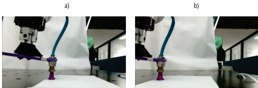
Figura 12. a) Primer punto para la matriz extrínseca, cámara izquierda; b) primer punto para la matriz extrínseca, cámara derecha
