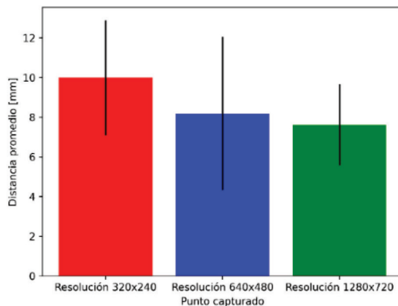
Figura 19. Distancia promedio. Valor de la pieza obtenido vs valor convencionalmente verdadero
