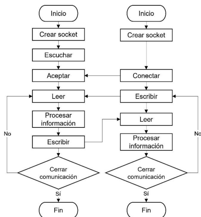
Figura 9. Diagrama de flujo de la comunicación socket
