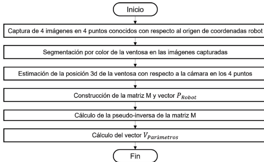
Figura 11. Diagrama de flujo del algoritmo que calcula la matriz extrínseca de la cámara
