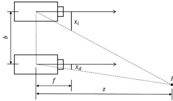
Figura 6. Geometría estéreo
