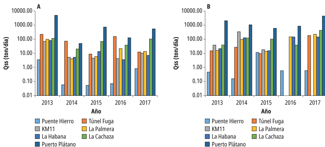
Figura 11. Cargas de sedimento en suspensión (Qss): a) primer semestre y b) segundo semestre
