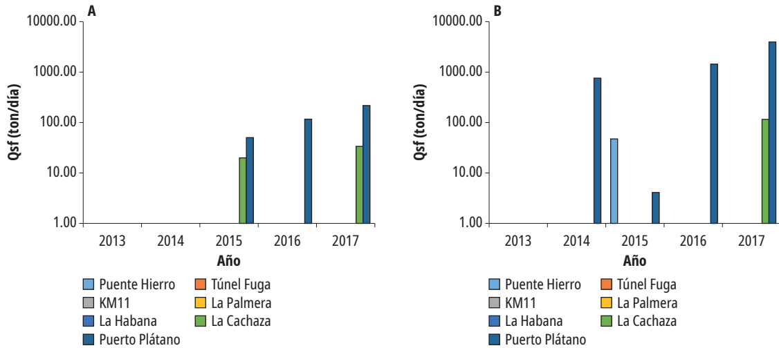
Figura 12. Cargas de sedimento de fondo (Qsf): primer semestre (a izquierda) y segundo semestre (a derecha)
