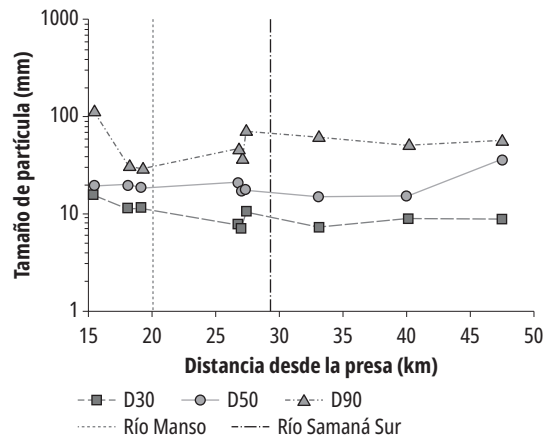
Figura 10. Variación del tamaño de partícula del lecho
