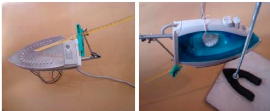
FIGURA 7 Posiciones de la plancha para mostrar la acción de la convección. En ambas situaciones se conserva la posición relativa del termómetro respecto de la base.
