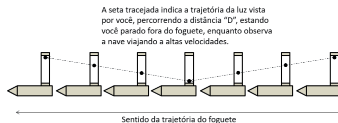
Figura 3. Trajetória da luz – situação 2.
