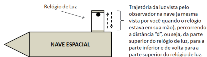
Figura 2. Trajetória da luz – situação 1.
