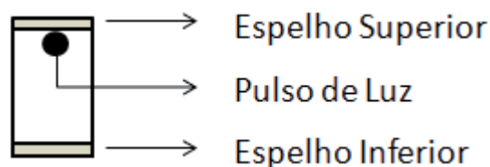
Figura 1. Relógio de luz.
