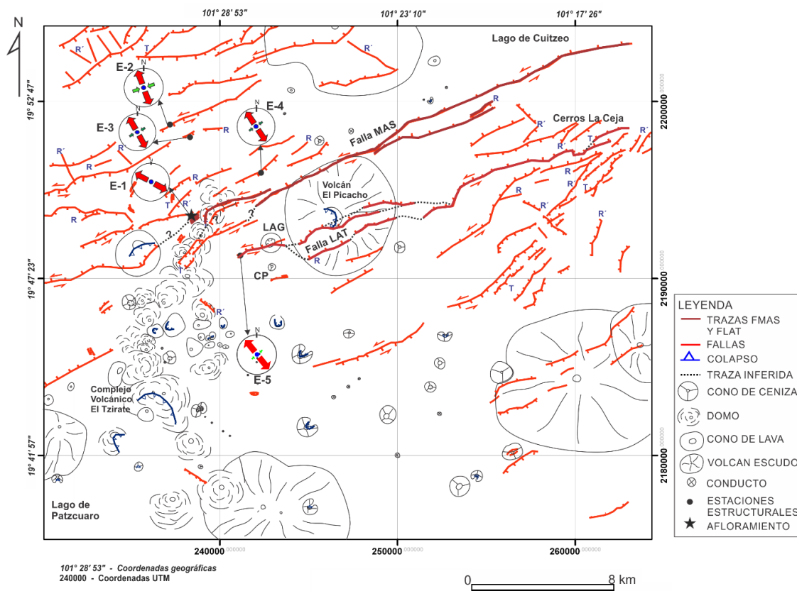
Figura 4 Mapa estructural de la región de estudio resaltando las trazas de las fallas El Malpaso-El Salto y La Alberca-Teremendo, así como las estructuras de alto y bajo ángulo (estructuras de relev). Las fallas indican el campo de esfuerzos actual en la región (Modificada de Pérez-Orozco et al. , 2018).
