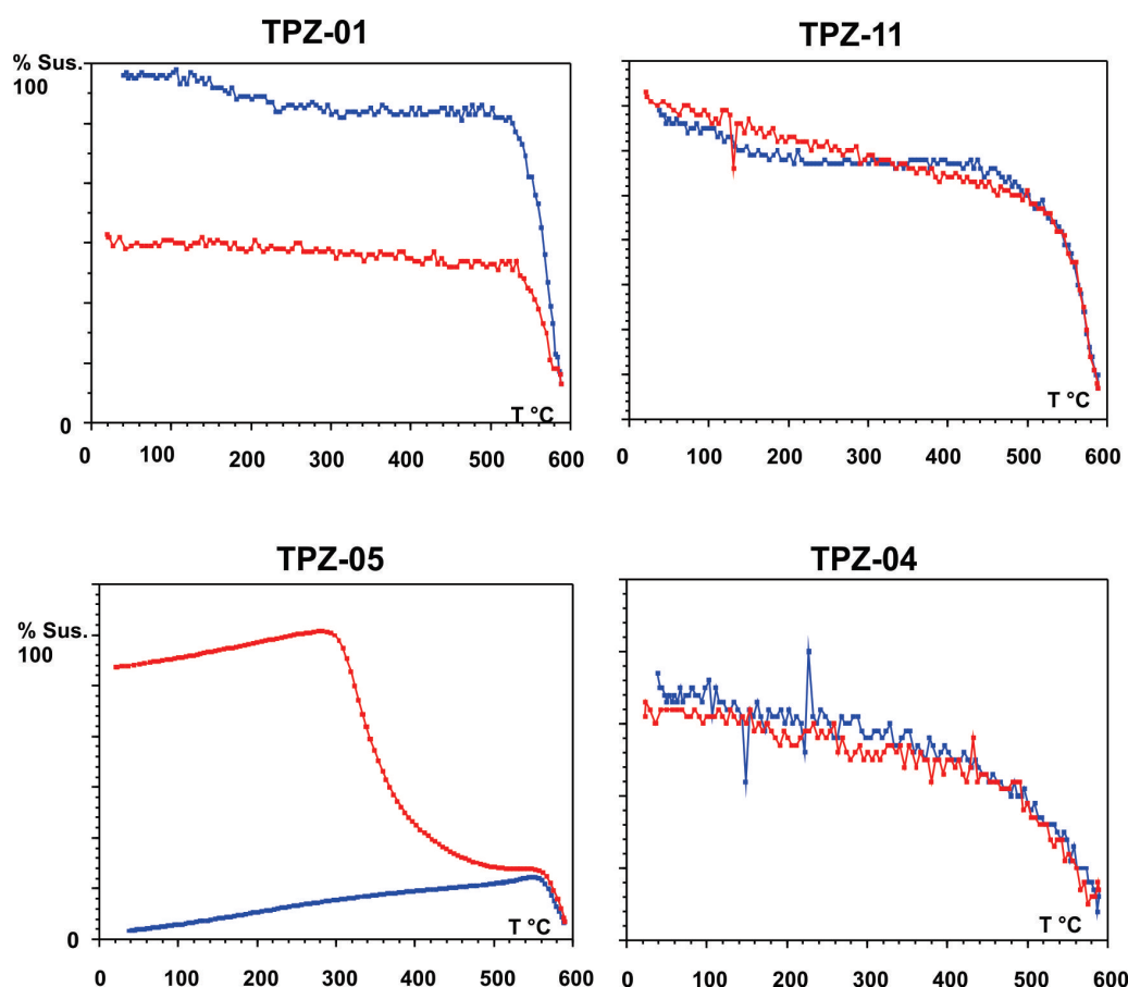
Figura 2 Curvas representativas de susceptibilidad vs temperatura (K-T). La línea roja indica el comportamiento de la susceptibilidad durante el calentamiento y la línea azul durante el enfriamiento. La susceptibilidad relativa se indica en unidades arbitrarias.
