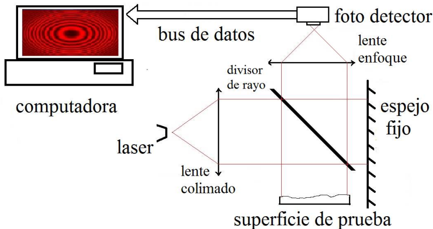
FIGURA 1 Interferómetro Twyman-Green
