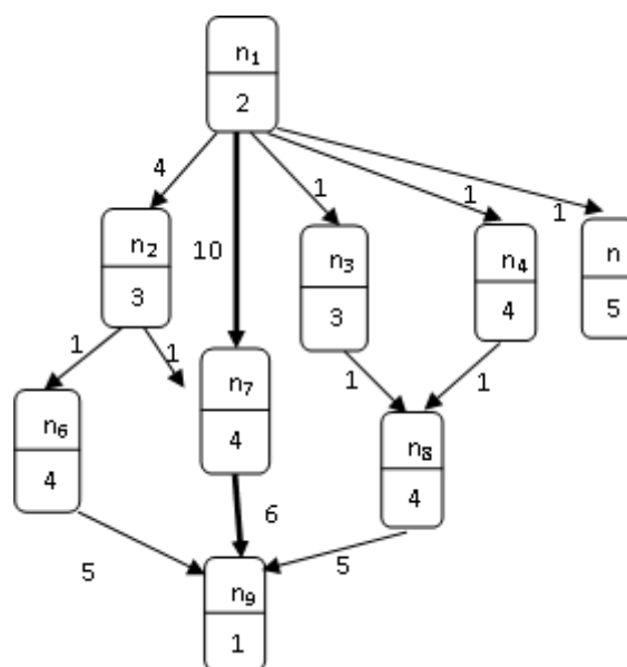
FIGURA 1 Grafo dirigido acíclico de una tarea [6].
