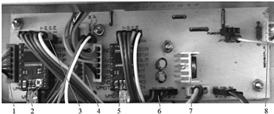
FIGURA 12. Tarjeta de control desarrollada.
