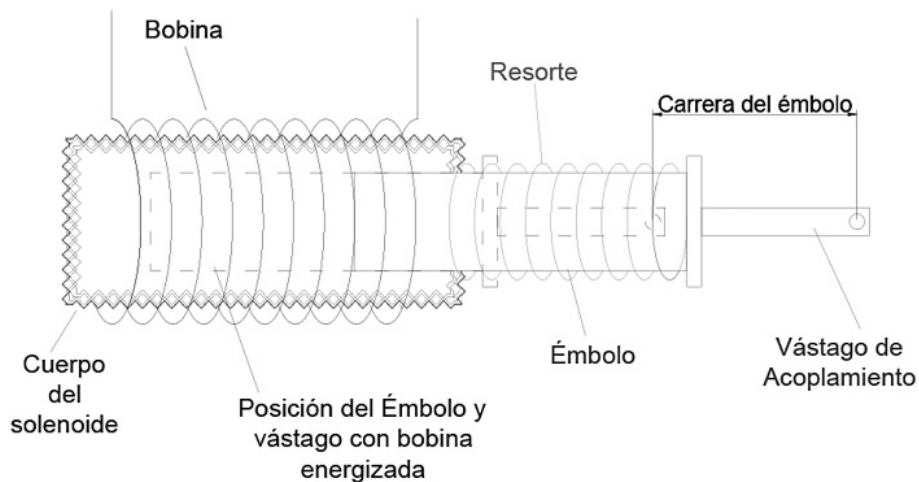
FIGURA 10. Solenoide
