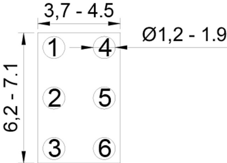
FIGURA 5. Matriz o carácter generador (mm)
