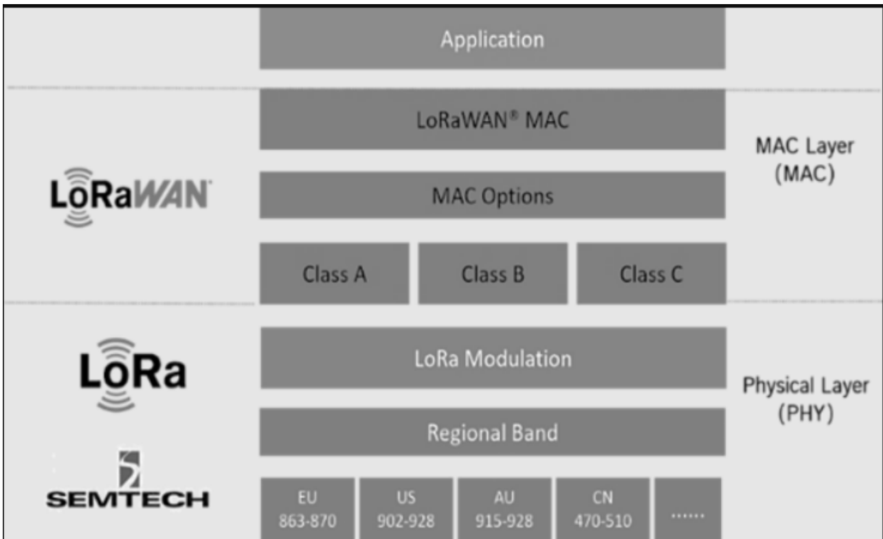
Figura 5. Pila de protocolos Lora. Fuente: [11].
