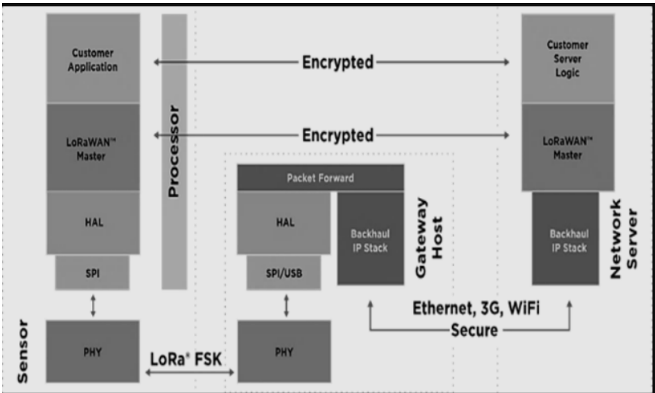
Figura 4. Especificación LoRaWAN. Fuente: [10]
