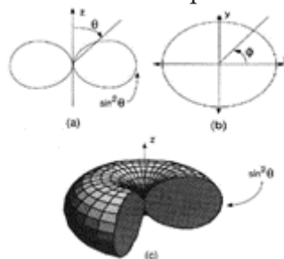
Figura 8. Patrón de radiación para una antena omnidireccional. (a) Elevación de un dipolo genérico, (b) Patrón de azimuth de un dipolo genérico (c) Patrón de radiación 3D. Fuente: [20].
