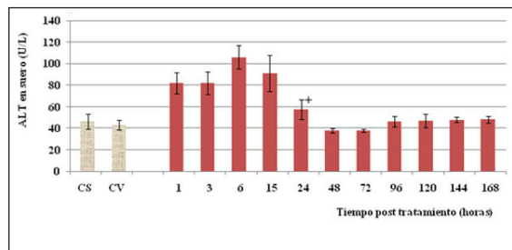
FIGURA 3. DETERMINACIÓN DE LA ACTIVIDAD DE LA ENZIMA ALT EN SUERO DE RATONES TRATADOS CON VENENO DE Bothrops colombiensis (Paracotos - Edo. Miranda).
