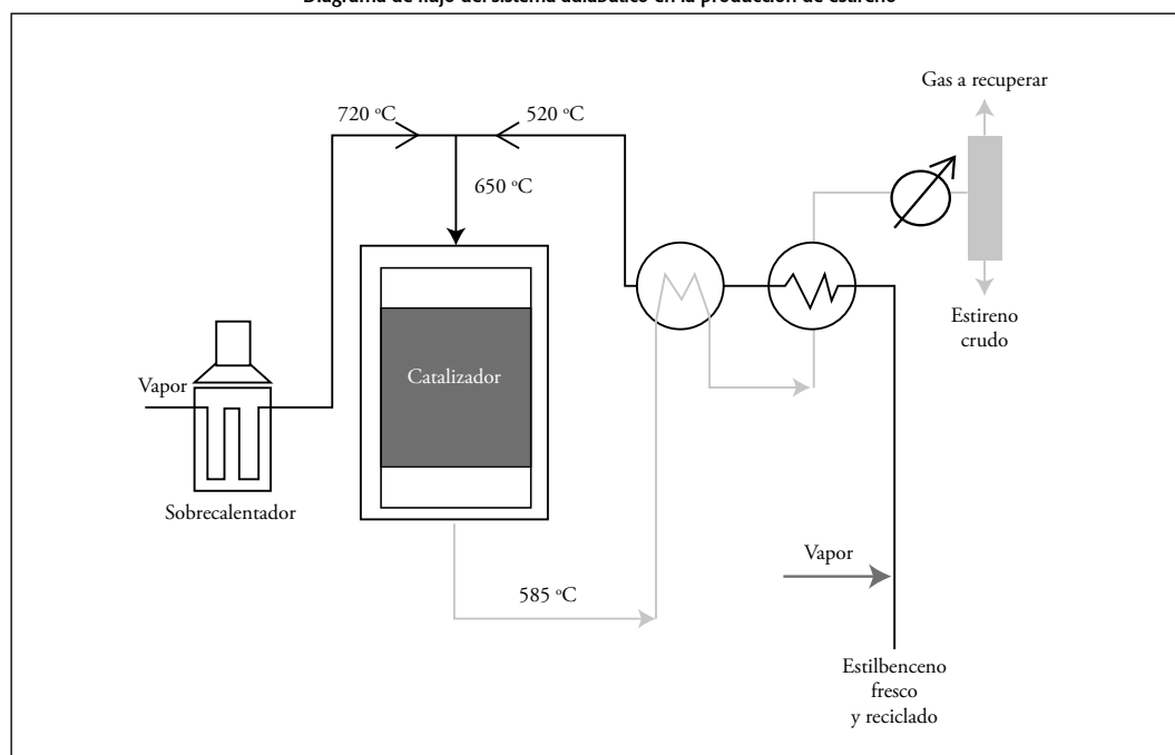
Figura 2 Diagrama de flujo del sistema adiabático en la producción de estireno
