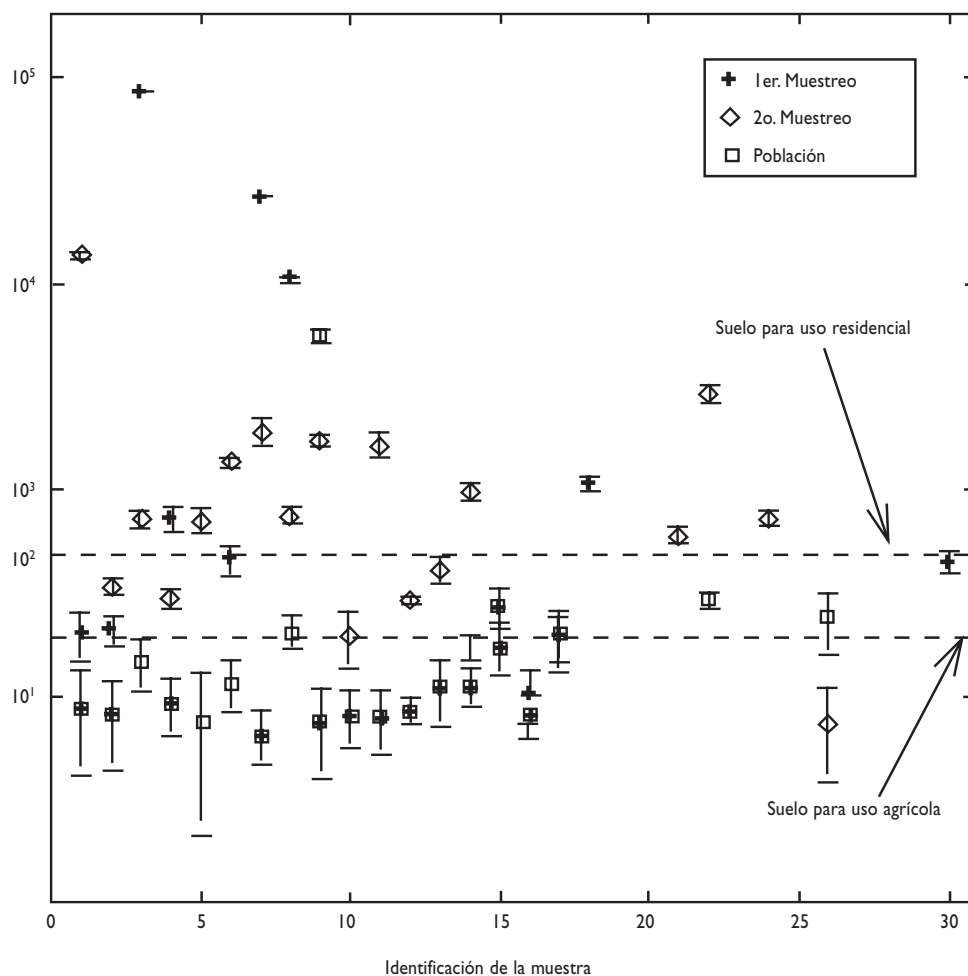
FIGURA 4. CONCENTRACIÓN DE Pb EN SUELO DE LOS TERRENOS, DE AGOSTADERO Y CULTIVO, LOCALIZADOS EN TORNO A LA RECICLADORA, ASÍ COMO DEL POBLADO DE SAN IGNACIO, FRESNILLO ZACATECAS. SE MUESTRAN DOS LÍNEAS QUE INDICAN LOS LÍMITES ESTABLECIDOS PARA EL USO DEL SUELO. LAS MUESTRAS SE TOMARON EN LOS MESES DE ENERO Y ABRIL DE 2005
