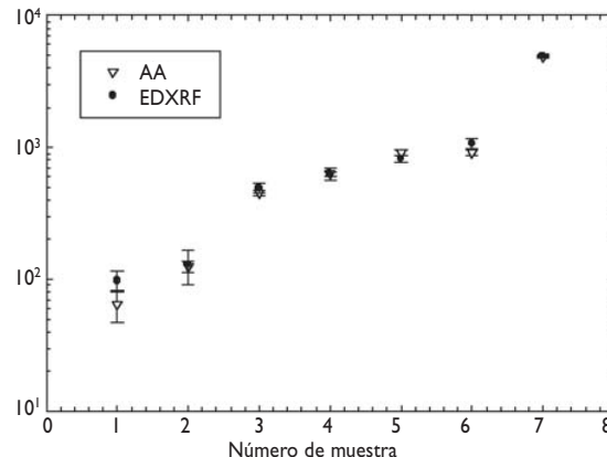
FIGURA 2. CONCENTRACIÓN DE Pb EN SIETE MUESTRAS DETERMINADA POR ABSORCIÓN ATÓMICA CON HORNO DE GRAFITO (AA) Y POR ENERGÍA DISPERSA DE FLUORESCENCIA DE RAYOS X (EDXRF), SAN IGNACIO, ZACATECAS
