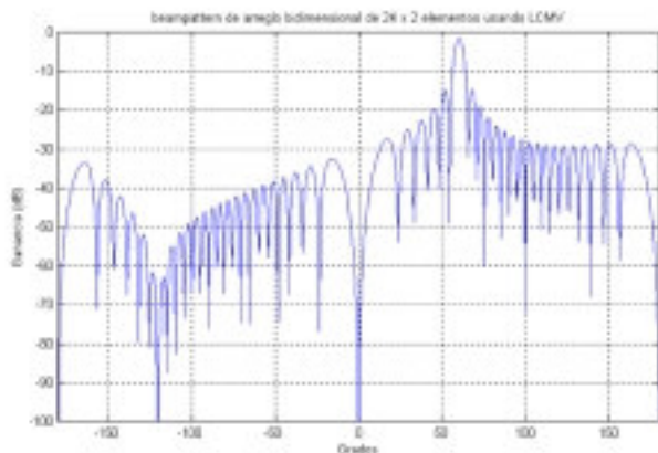
Fig. 20 Pattern azimutal dirigido a 60° del arreglo 24 x 2 usando LCMV.
