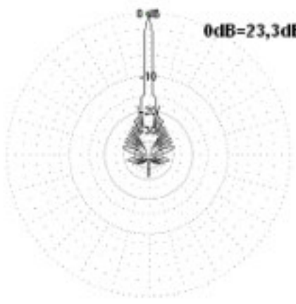
Fig. 11 Pattern de radiación de un arreglo bidimensional de 24 x 2 (monopolos de 0,25λ) con separación de 0,5λ y 0,25λ en X e Y, respectivamente.
