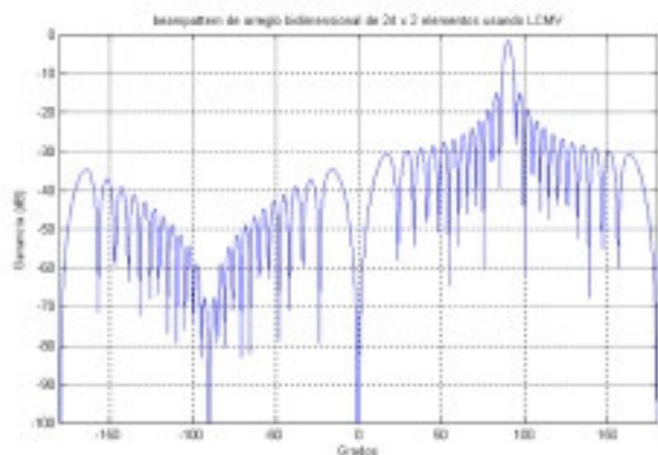
Fig. 19 Pattern azimutal dirigido a 90° (broadside) del arreglo 24 x 2 usando LCMV.
