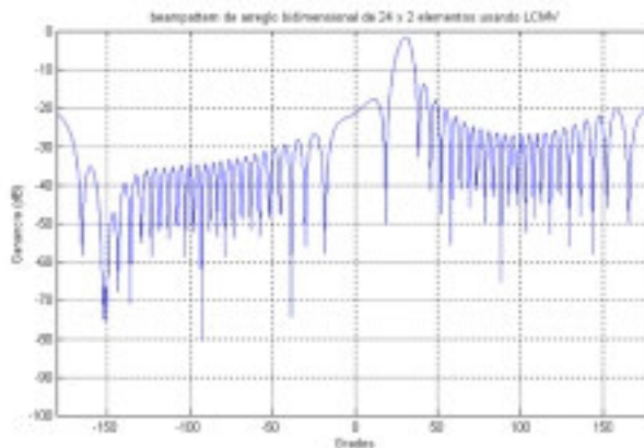
Fig. 21 Pattern azimutal dirigido a 30° del arreglo 24 x 2 usando LCMV.
