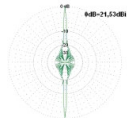
Fig. 9 Diagrama de radiación horizontal de un arreglo lineal 32 x 1 Broadside (monopolos de 0,25\lambda ) separados 0,5\lambda .
