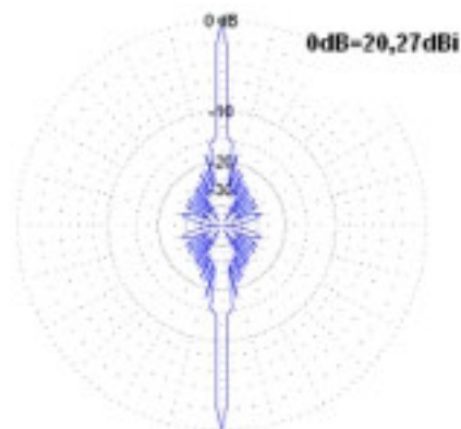
Fig. 5 Diagrama de radiación horizontal de un arreglo lineal 24 x 1 Broadside (monopolos de 0,25\lambda ) separados 0,5\lambda .
