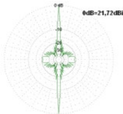
Fig. 6 Diagrama de radiación horizontal de un arreglo lineal 24 x 1 Broadside (monopolos de 0,25\lambda ) separados 0,75\lambda .
