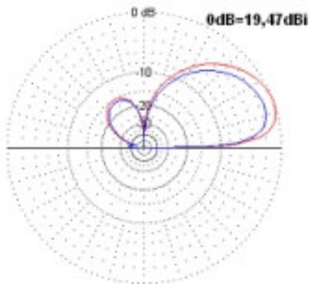
Fig. 14 Pattern de radiación vertical del arreglo 24 x 2 para tierra húmeda ( \epsilon_r=30 \sigma=0,02 \Omega^{-1}/m ) sin radiales (azul) y con radiales (rojo).
