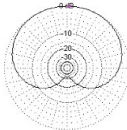
Fig. 10 Diagrama de radiación de 2 monopolos de 0,25λ separados 0,25λ y en cuadratura de fase.
