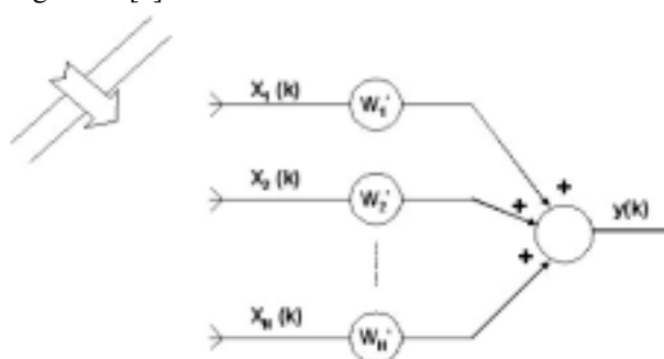
Fig. 15 Esquema de un beamformer.
