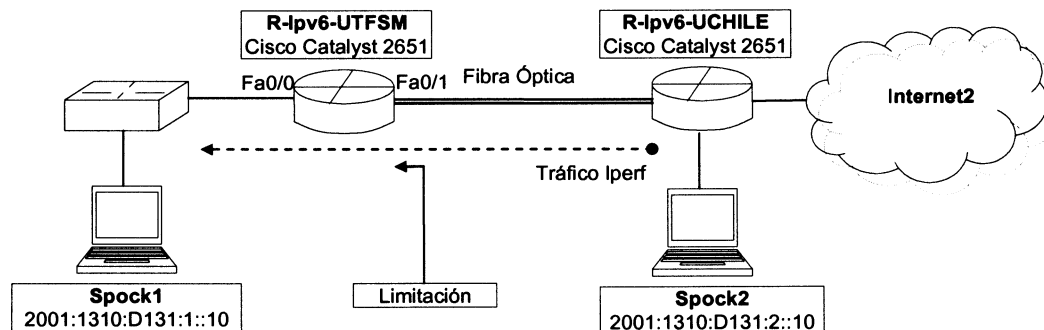
Fig. 3 Diagrama de Medición de Tráfico Multimedial.
