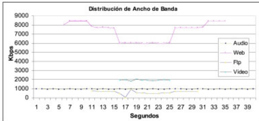
Gráfico 1 Distribución de Ancho de Banda.
