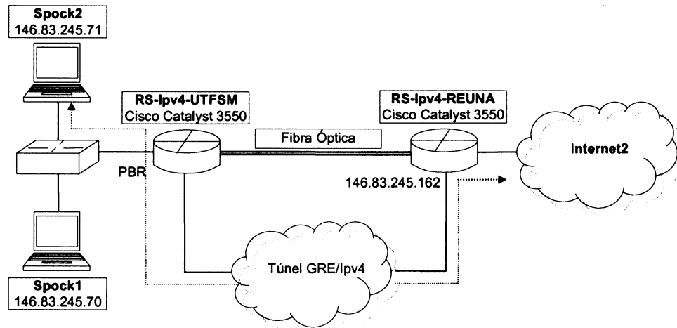
Fig. 1 Diagrama de medición para PBR.
