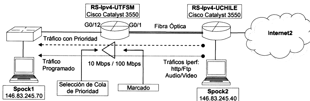
Fig. 2 Diagrama de Medición de Tráfico Multimedial.
