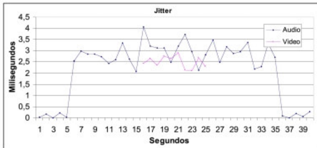
Gráfico 2 Distribución de Jitter.
