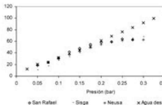
Figura 12. Flujo de permeado bajo diferentes presiones. Agua cruda con CAP. San Rafael, CAP = 25mg/L; Sigga, CAP = 30mg/L; Neusa, PAC = 22 mg/L
