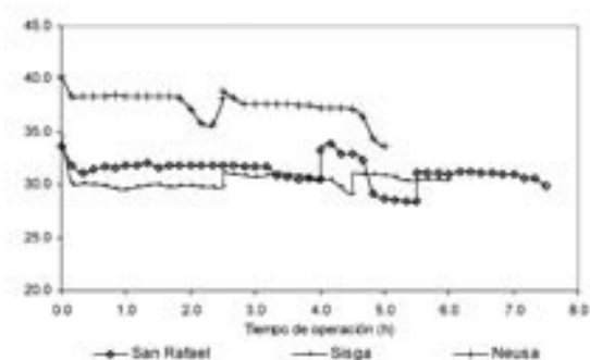
Figura 13. Variación del flujo en función del tiempo. SanRafael, P=0.125 bar, CO=3.48 mg C/L, CAP 25 mg/L; Sigga P=0.125 bar, COT=4.33 mg C/L, CAP 30 mg/L; Neusa, P=0.15 bar, COT=4.2 mg/L, CAP 22 mg/L
