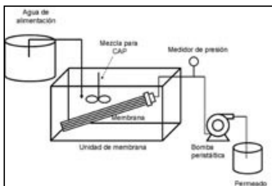
Figura 1. Diagrama sistema de MF
