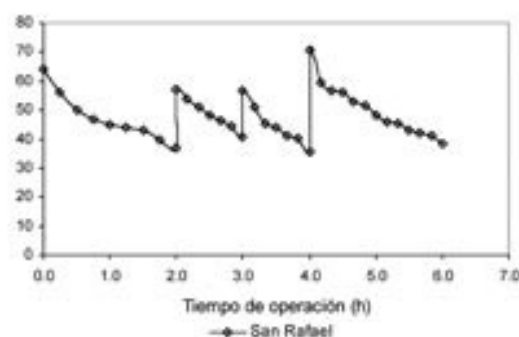
Figura 4. Variación del flujo en función del tiempo.
