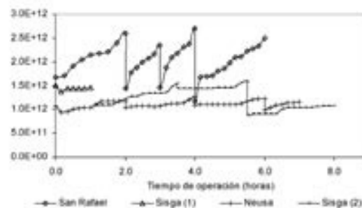
Figura 6. Resistencia total proporcionada por la membrana y materiales colmatantes
