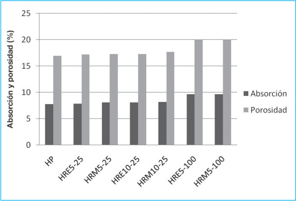
Figura 8. Absorción y porosidad de los hormigones
