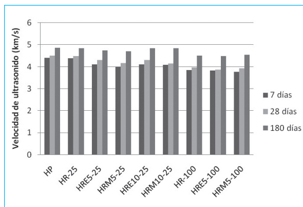
Figura 4. Velocidad de ultrasonido en los hormigones
