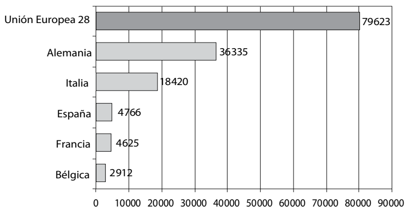
GRÁFICA 9. Capacidad eléctrica en energía solar fotovoltaica (KTP) de los cinco mayores productores de la Unión Europea-28 en 2013
