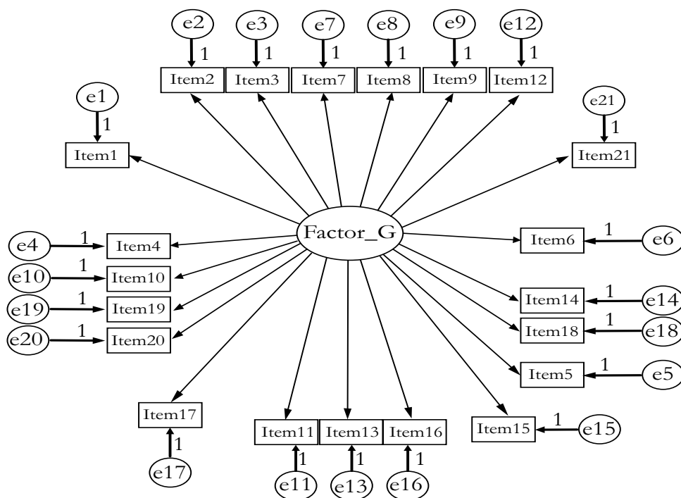
Figura 1. Representación gráfica del modelo factorial del instrumento de actitudes hacia las matemáticas
