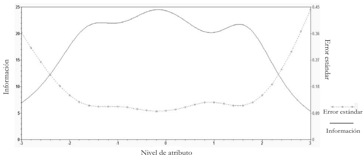
Figura 2. Función de información y error estándar para el test
