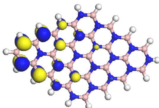
Figura 2b. Orbital molecular HOMO del h-BN 1,0 nm 2 , cuya contribución atómica se tiene por parte de los orbitales 2p z del nitrógeno.
