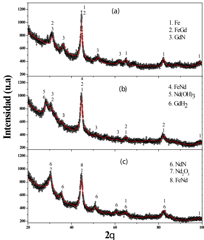
Figura 1. Patrones de difracción de rayos X de las muestras (a) \text{Gd}_{0.257-x}\text{Fe}_{0.743} , (b) \text{Gd}_{0.1285}\text{Nd}_{0.1285}\text{Fe}_{0.743} y (c) \text{Nd}_{0.257}\text{Fe}_{0.743} con 72 horas de molienda
