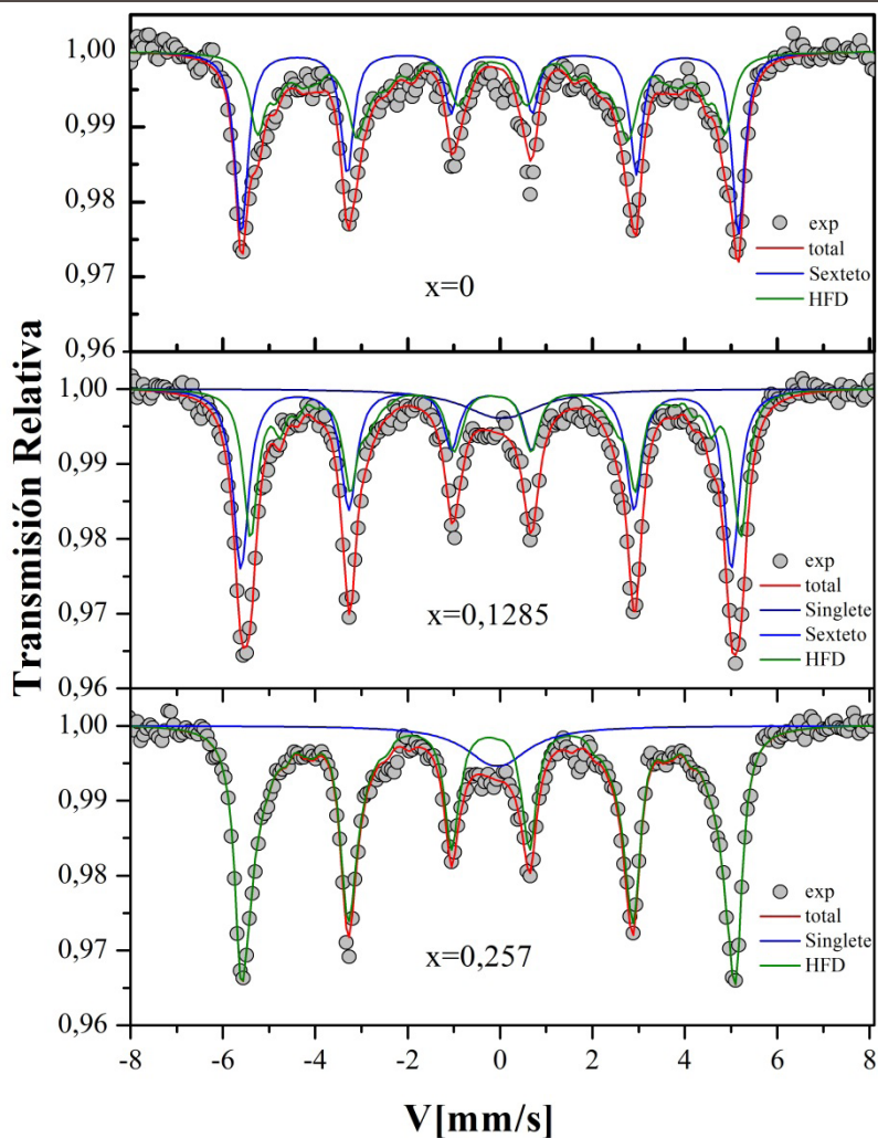
Figura 2. EM del sistema Gd_{0,257-x}Nd_xFe_{0,743} con x=0, 0,1285, 0,257 molido durante 72 horas
