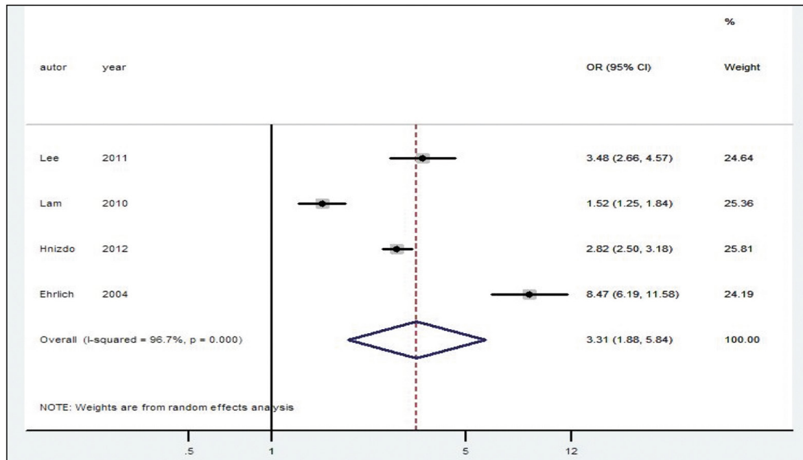
Figura 3. Foresplot.
