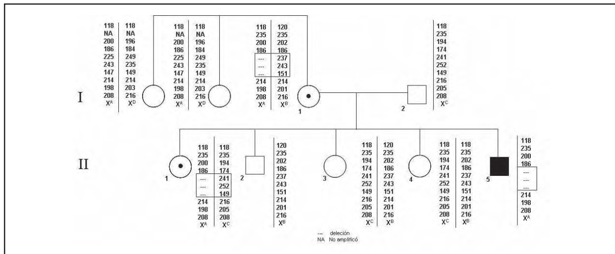
Figura 3. Genealogía y haplotipos familia DMD 108. Se muestra el haplotipo construido mediante STR del gen de la distrofia. X^A corresponde al haplotipo del afectado (haplotipo de riesgo), X^B corresponde al haplotipo no ligado a la mutación, --- indica deleción. Se observa que en las mujeres I.1 y II.1 hay pérdida de heterocigocidad para los STR implicados en la deleción (recuadro), II.3 y II.4 heredaron el cromosoma X^B de la madre no ligado a la mutación y el X^C normal del padre indicando su estado de no portadora.
