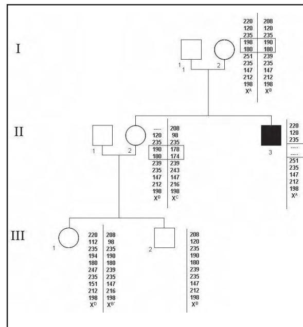
Figura 2. Genealogía y haplotipos familia DMD 7. Se muestra el haplotipo construido mediante STR del gen de la distrofia. X^A corresponde al haplotipo del afectado (haplotipo de riesgo), --- En II.3 indica la deleción en el afectado. El X^B corresponde al haplotipo no ligado a la mutación. Se observa que en las mujeres I.2 y II.2 no hay pérdida de heterocigocidad para los STR implicados en la deleción del afectado, lo cual se indica en el recuadro.
