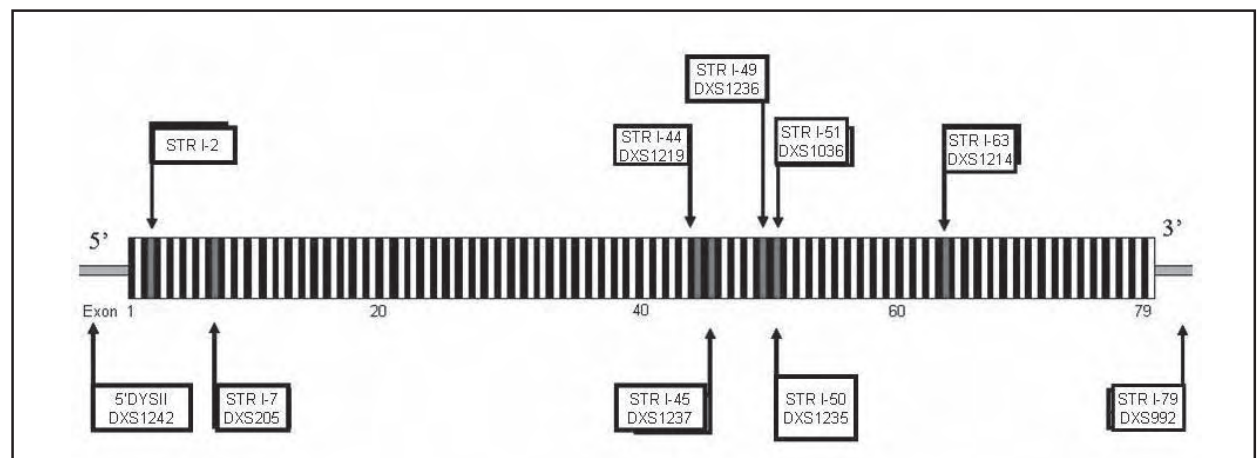
Figura 1. Distribución de los STRs analizados en el gen de la distrofina. Se analizaron ocho STRs intragénicos, distribuidos entre en intrón 2 (STR I-2) y 63 (STR I-63) del gen, así como dos STRs extragénicos, uno situado en el extremo 5' (DYSII) y el otro en el extremo 3' (STR I-79).
