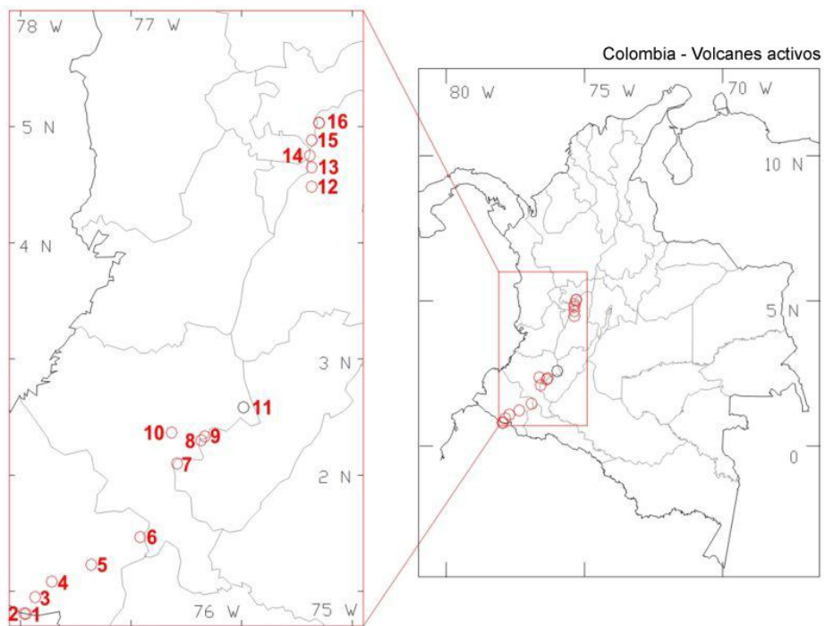
Figura 2. Mapa de localización de los principales volcanes activos en Colombia. Tomado de www.ingeminas.gov.co
