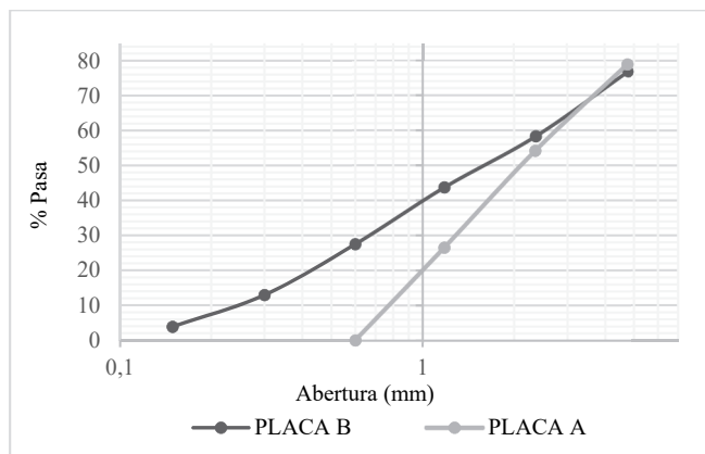
Figura 2. Distribución granulométrica de los agregados usados para las placas A y B.
