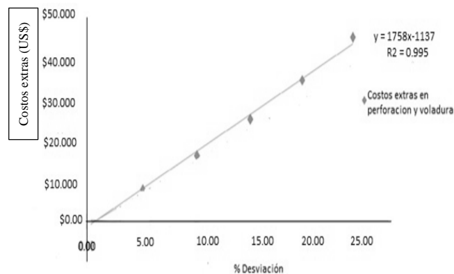
Figura 3. Costos extras en perforación y voladura y porcentaje de desviaciones (%).
