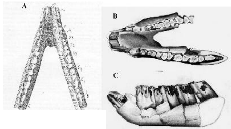
FIG. 2. A Reconstrucción idealizada de Anatrachytherus soriai gen. et sp. nov. (originalmente asignada a Trachytherus spegazzinianus Ameghino) realizada por Florentino Ameghino (1897, Fig. 13). B . Anatrachytherus soriai (holotipo, MACN A52-490), vista oclusal. C . Anatrachytherus soriai (holotipo, MACN A52-490), vista lateral izquierda. Escala: 1 cm.
