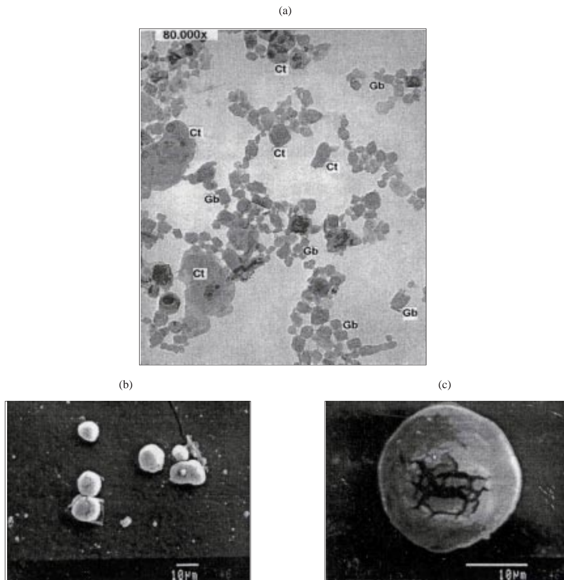
Figura 2. Micrografias de partículas de gibbsita do Latossolo Vermelho-Escuro (amostra 11) presentes nas frações argila (microscópio eletrônico de transmissão) (a) e silte (microscópio eletrônico de varredura) (b e c).
