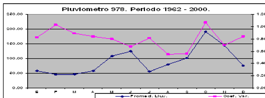
Fig # 4. Pluviómetro 978. La Siberia. Municipio Gibara. Periodo 1962-2000
