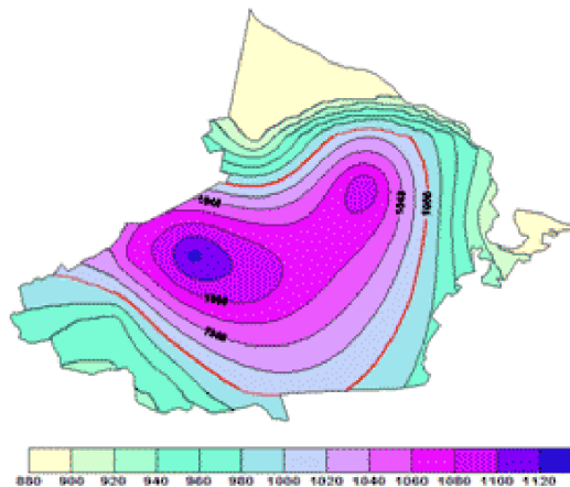
Fig. # 5 Mapa Isoyetico Hiperanual Municipio Gibara (Periodo 1978-2007)
