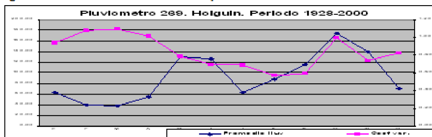
Fig # 3. Pluviómetro 269. Iberia. Municipio Gibara. Periodo 1928-2000
