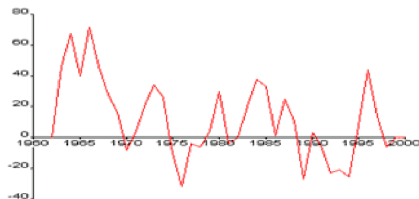
Graf. # 2 Prueba de Pettit. Pluviómetro 978. La Siberia. Municipio Gibara
