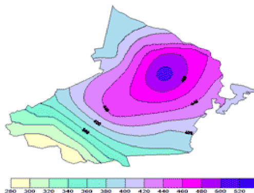
Fig # 6 Mapa Isoyetico Periodo Poco Lluvioso Municipio Gibara (Periodo 1978-2007)
