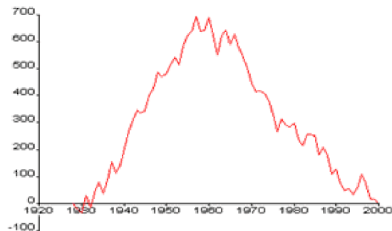
Graf. # 1. Prueba de Pettit. Pluviómetro 269 "Iberia". Municipio Gibara
