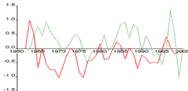
Graf. # 4 Prueba de Mann.
