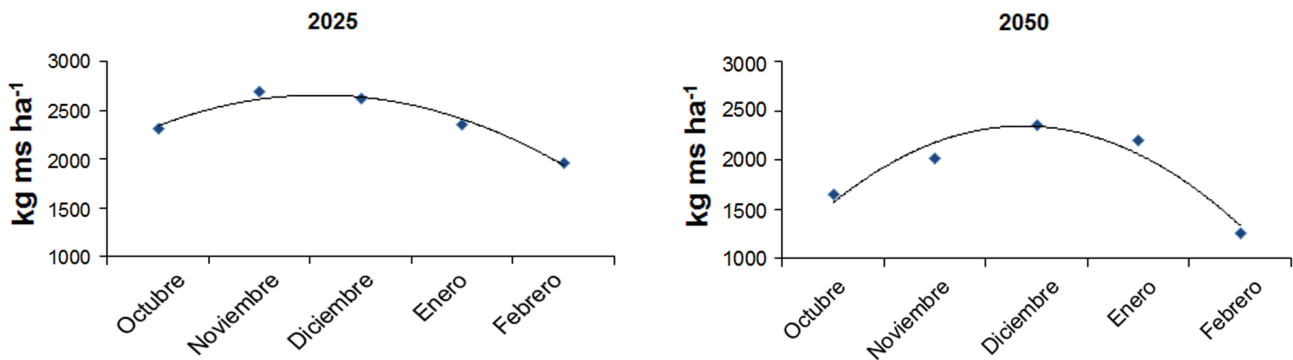
Figura 4. Rendimientos simulados en el cultivo del trigo en fechas de siembra mensuales en Tapaste
