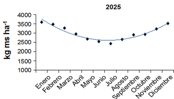
Figura 1. Rendimientos simulados en el cultivo del arroz en fechas de siembra mensuales en Los Palacios
