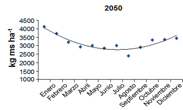
Figura 2. Rendimientos simulados en el cultivo del maíz en fechas de siembra mensuales en Tapaste
