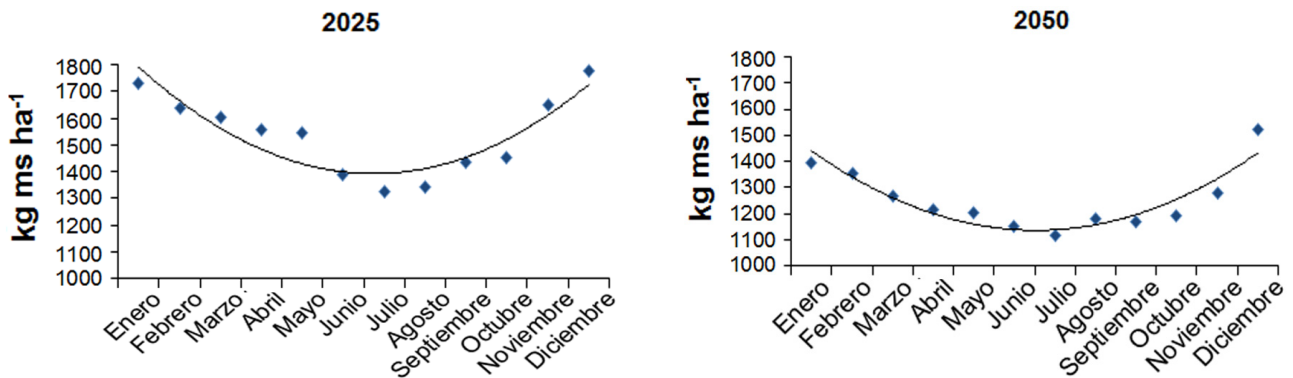
Figura 3. Rendimientos simulados en el cultivo del sorgo en fechas de siembra mensuales en Guantánamo
