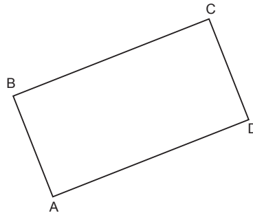
Figura 1. Rectángulo \square ABCD
