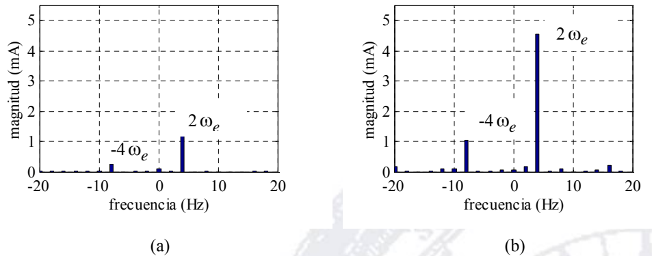
Figura 6: Armónicos inducidos por saturación. a) Armónicos de la corriente portadora de secuencia negativa, en coordenadas de secuencia negativa, para un motor de ranuras abiertas. B) para un motor de ranuras cerradas. |i_{qds}|=2 A, \omega_e=2 Hz, \omega_r=1 Hz, V_c=5 V y \omega_c=500 Hz. Motor #4 con rotor #2 y #1 respectivamente.
