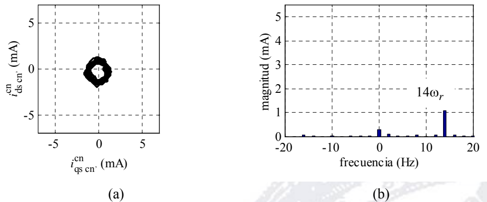
Figura 3: Corriente portadora de secuencia negativa, en coordenadas de secuencia negativa del motor #2 (S=36,R=28). Inversor lineal con |i_{qds}|=0 A, \omega_r=1 Hz, V_c=5 V y \omega_c=500 Hz a) Trayectoria y b) FFT de la corriente portadora de secuencia negativa.
