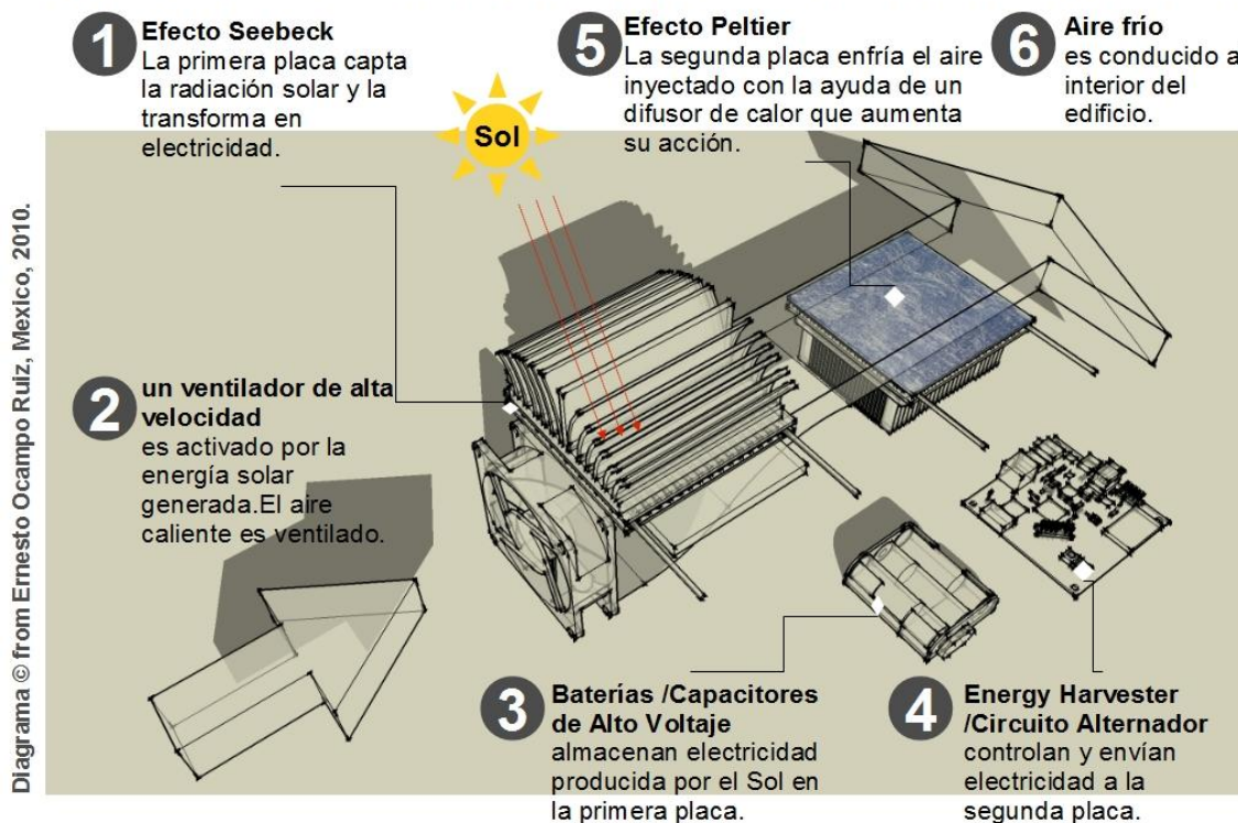
Figura 5. Esquema de funcionamiento del prototipo de enfriamiento termoeléctrico solar, desarrollo tecnológico y arquitectónico que trasforma el calor del Sol directamente en aire frío manipulando los efectos termoeléctricos Seebeck y Peltier de ciertos materiales constructivos y tecnologías de punta.
