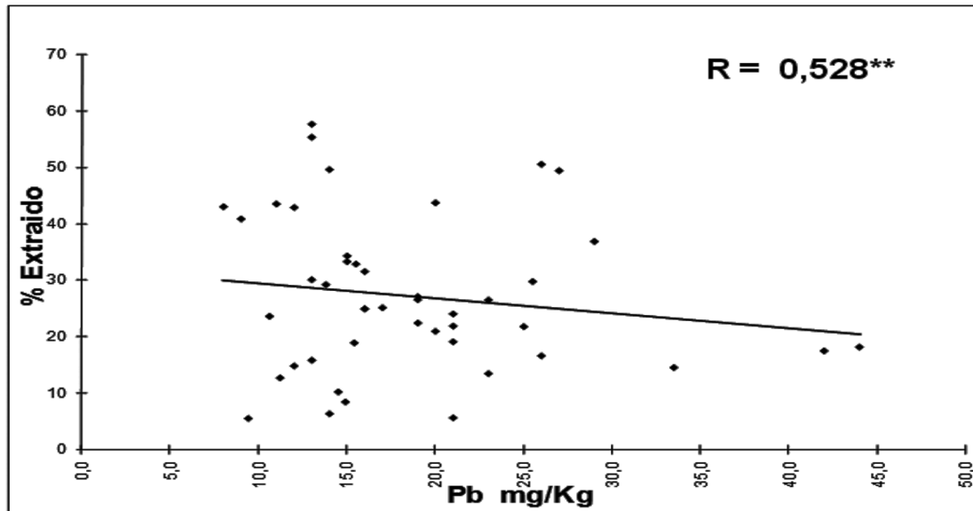
Figura 2. Cantidad de Pb extraído con EDTA-AcA, respecto a su contenido seudototal
