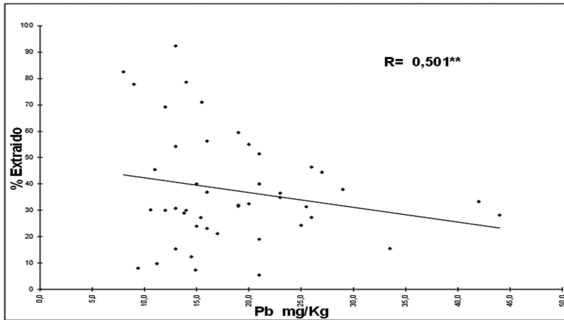
Figura 1. Cantidad de Pb extraído con pirofosfato alcalino respecto a su contenido seudototal
